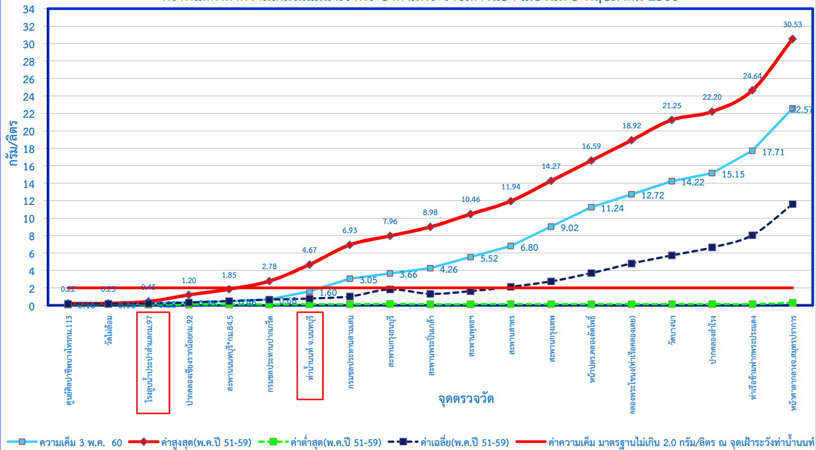
กราฟแสดงค่าความเค็มในแม่น้ำเจ้าพระยาตามพระราชเสาวนีย์ฯ เมื่อวันที่ 3 พฤษภาคม 2560
