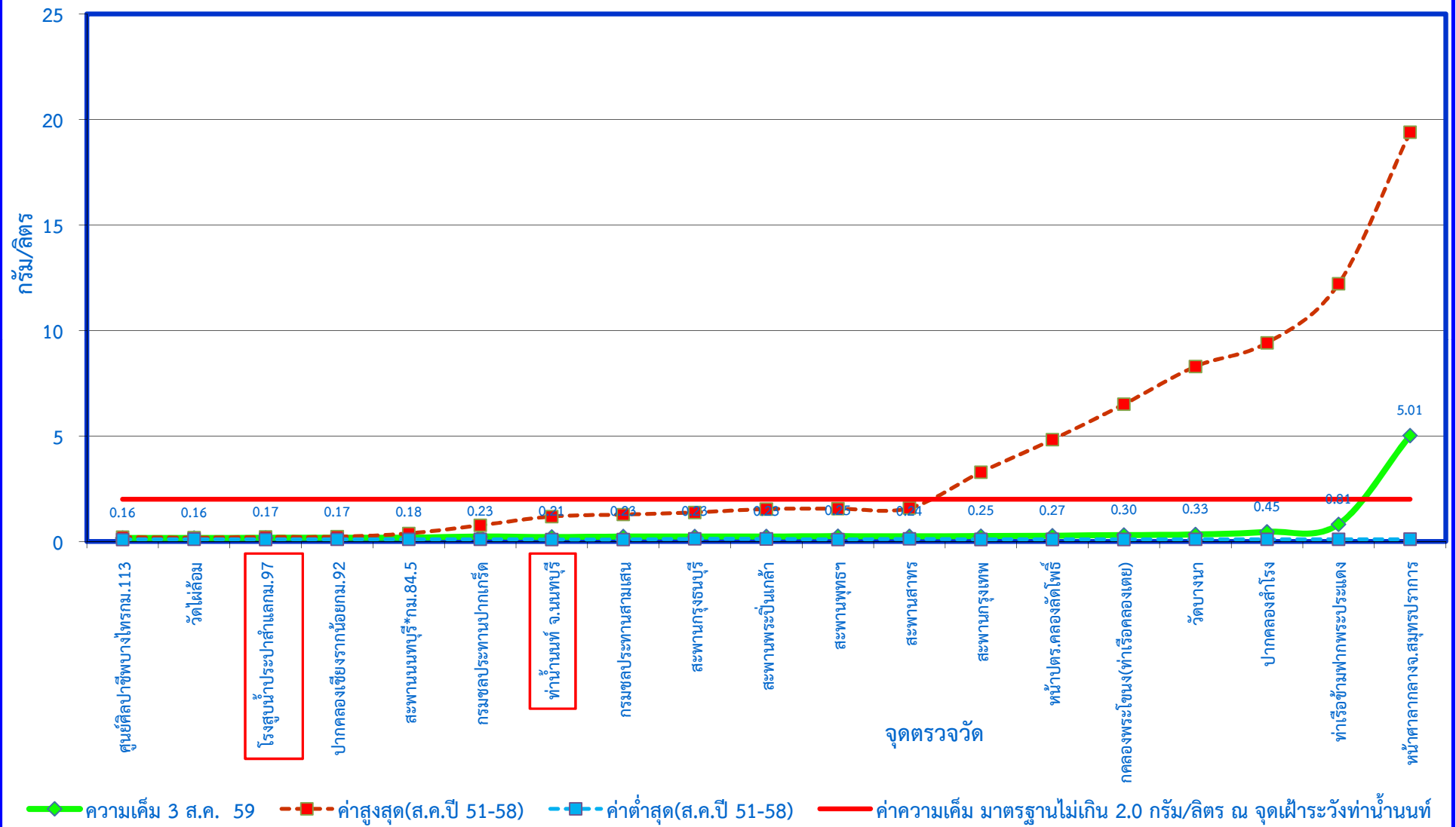
กราฟแสดงค่าความเค็มในแม่น้ำเจ้าพระยาตามพระราชเสาวนีย์ฯ เมื่อวันที่ 3 สิงหาคม 2559
