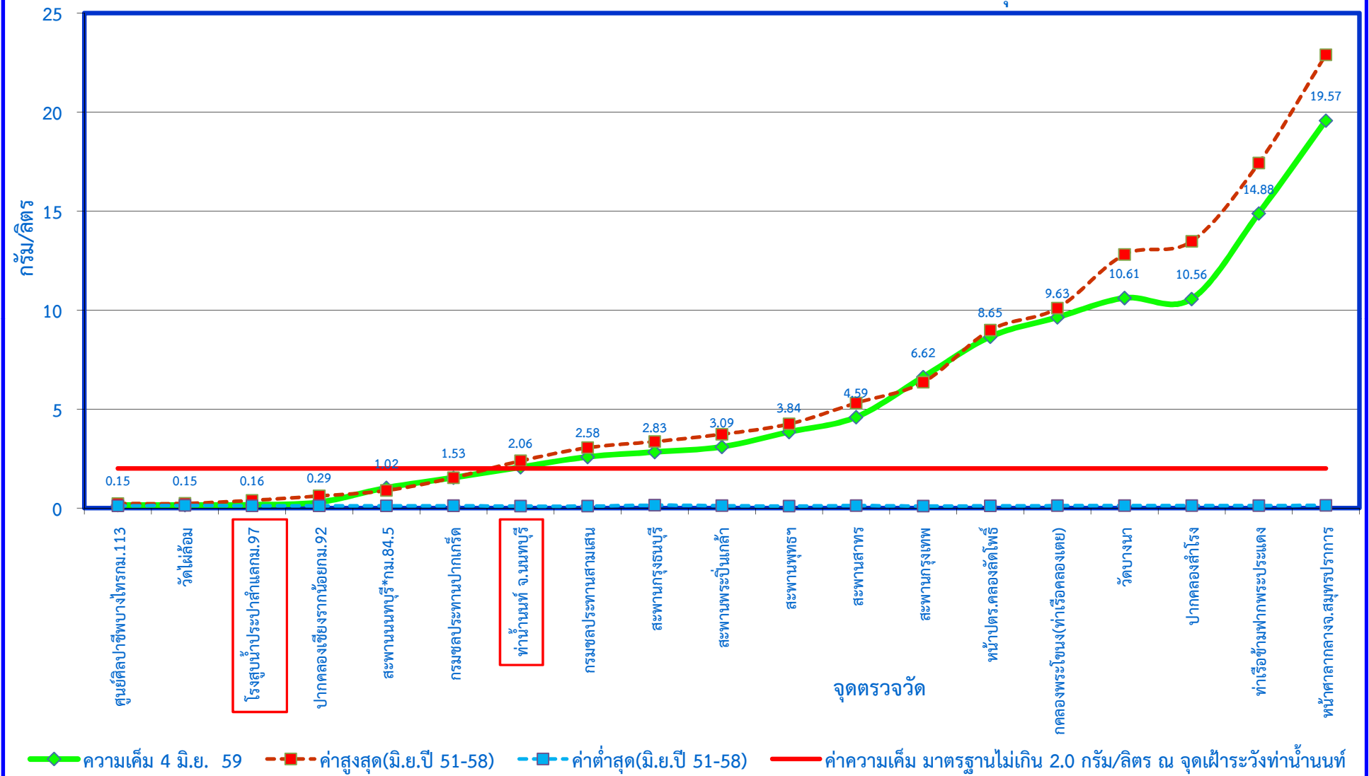
กราฟแสดงค่าความเค็มในแม่น้ำเจ้าพระยาตามพระราชเสาวนีย์ฯ เมื่อวันที่ 4 มิถุนายน 2559
