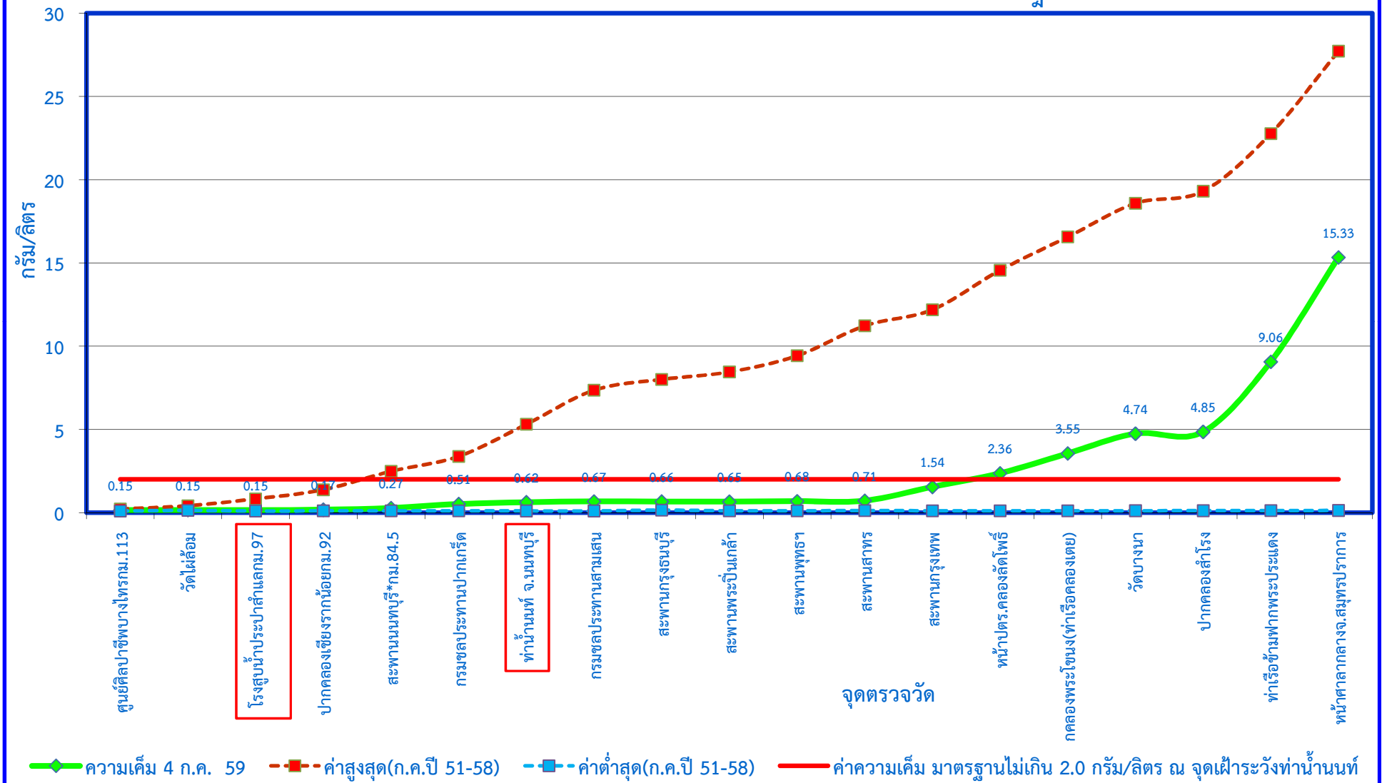
กราฟแสดงค่าความเค็มในแม่น้ำเจ้าพระยาตามพระราชเสาวนีย์ฯ เมื่อวันที่ 4 กรกฎาคม 2559
