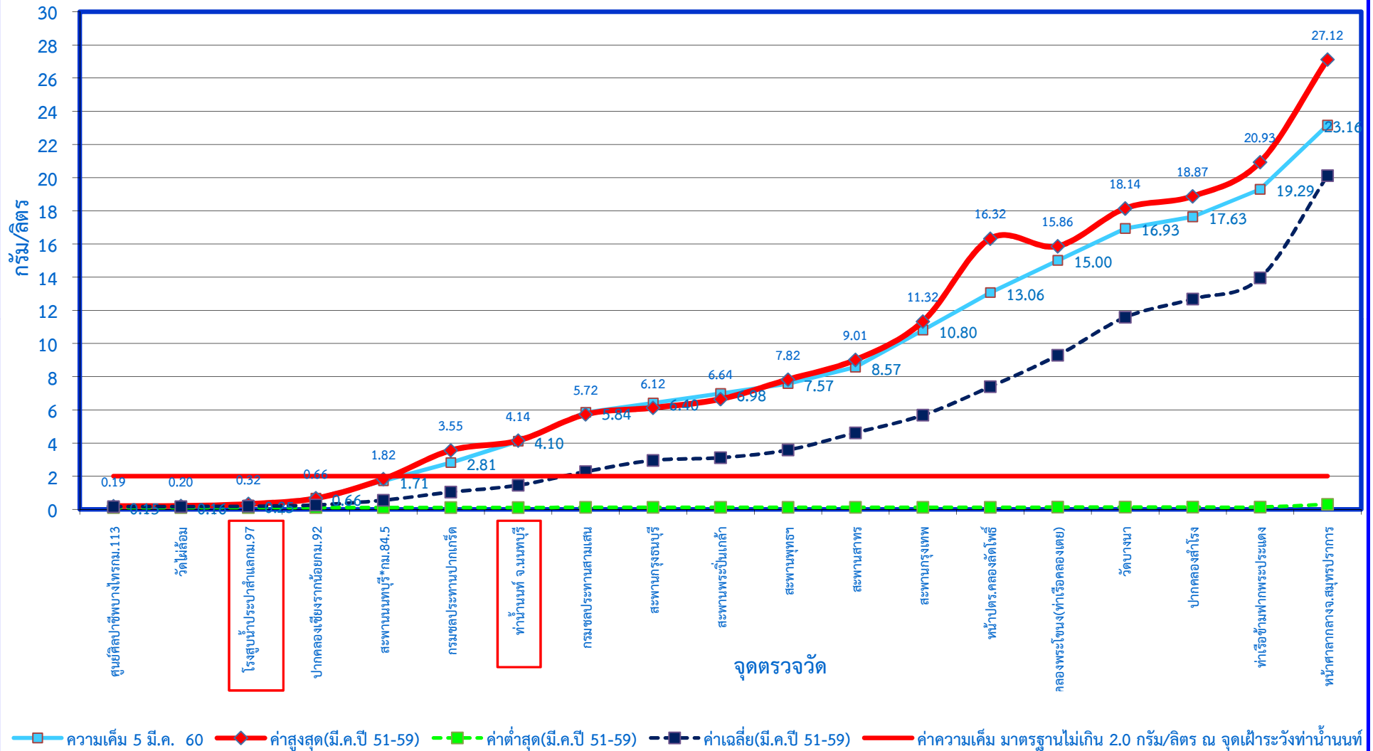
กราฟแสดงค่าความเค็มในแม่น้ำเจ้าพระยาตามพระราชเสาวนีย์ฯ เมื่อวันที่ 5 มีนาคม 2560
