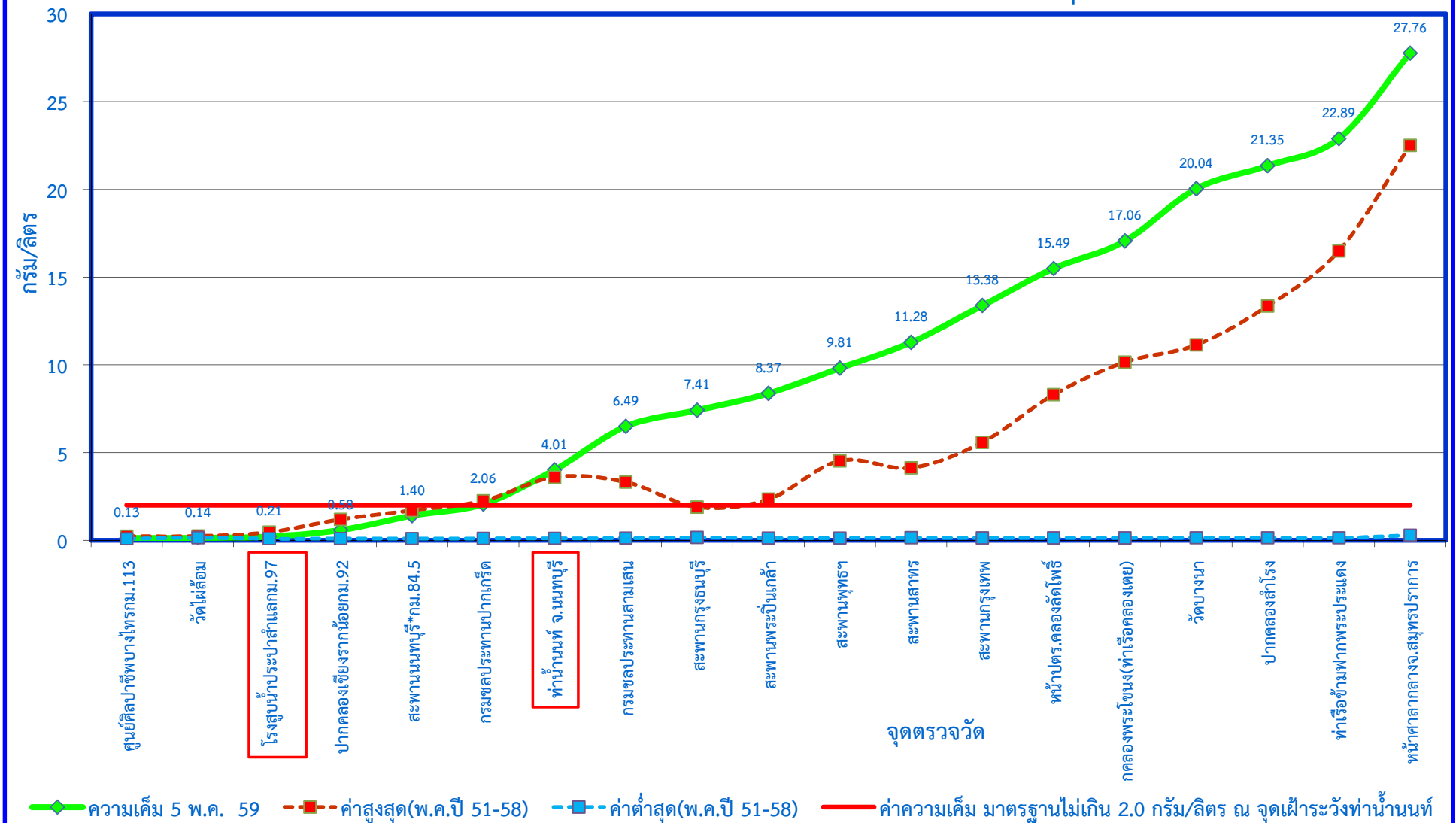
กราฟแสดงค่าความเค็มในแม่น้ำเจ้าพระยาตามพระราชเสาวนีย์ฯ เมื่อวันที่ 5 พฤษภาคม 2559
