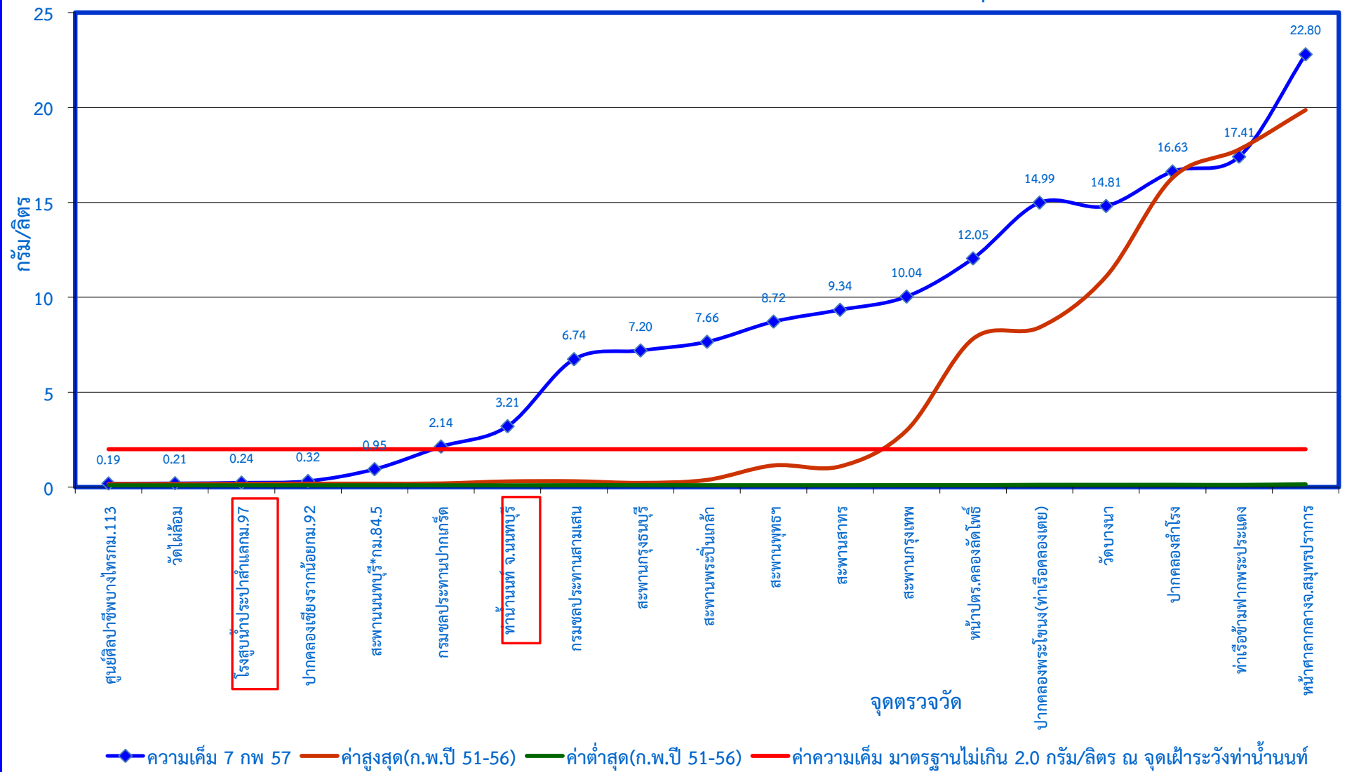
กราฟแสดงค่าความเค็มในแม่น้ำเจ้าพระยาตามพระราชเสาวนีย์ฯ เมื่อวันที่ ๗ กุมภาพันธ์ ๒๕๕๗
