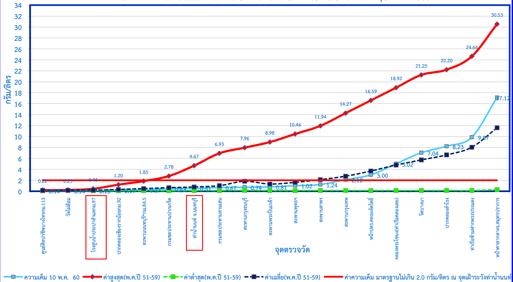
กราฟแสดงค่าความเค็มในแม่น้ำเจ้าพระยาตามพระราชเสาวนีย์ฯ เมื่อวันที่ 10 พฤษภาคม 2560
