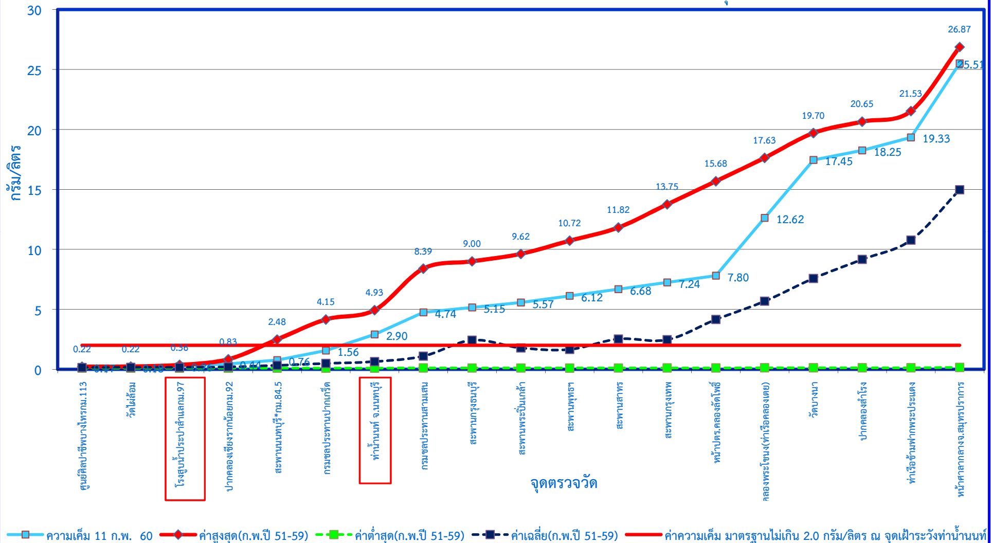
กราฟแสดงค่าความเค็มในแม่น้ำเจ้าพระยาตามพระราชเสาวนีย์ฯ เมื่อวันที่ 11 กุมภาพันธ์ 2560
