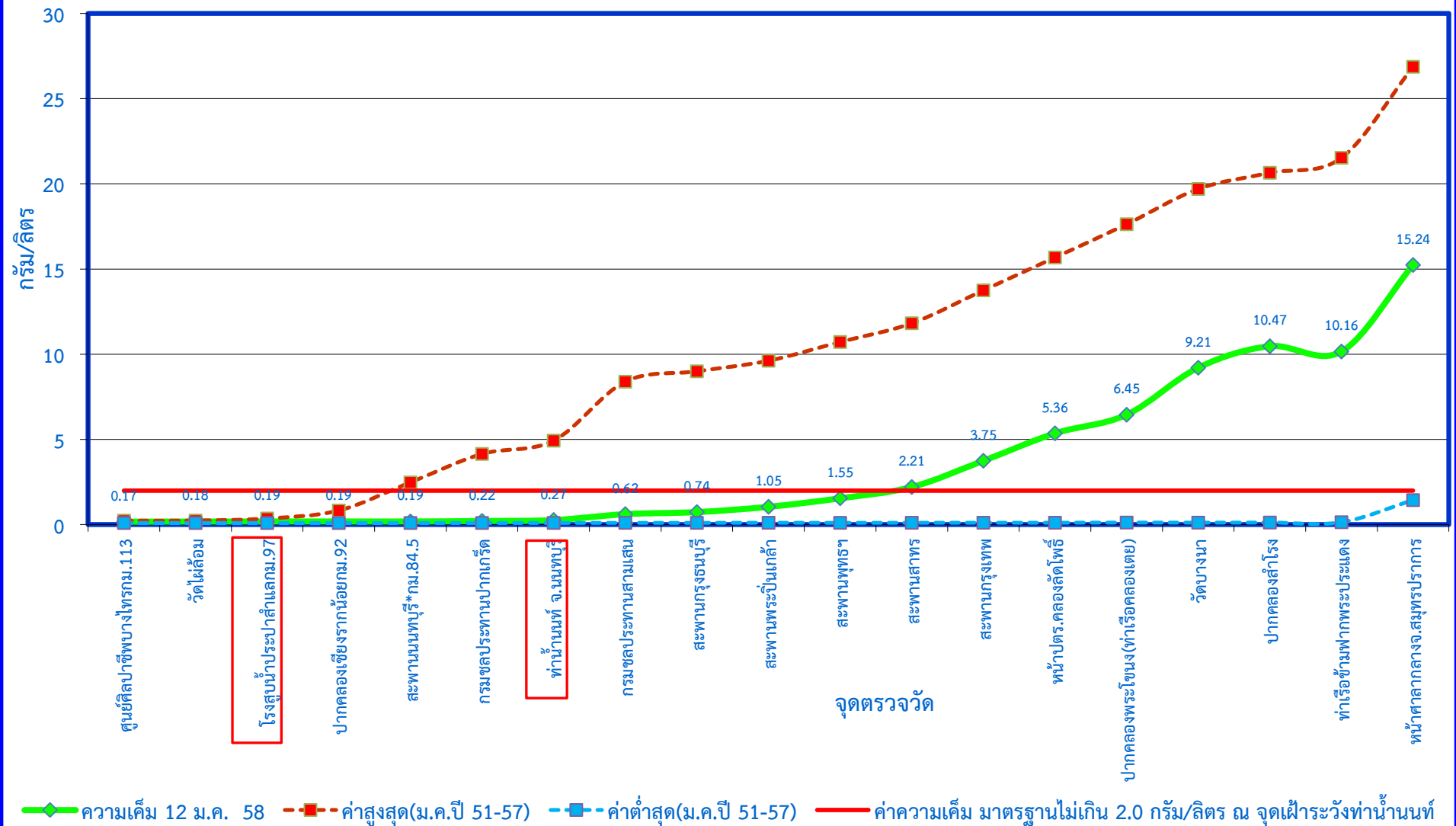
กราฟแสดงค่าความเค็มในแม่น้ำเจ้าพระยาตามพระราชเสาวนีย์ฯ เมื่อวันที่ 12 มกราคม 2558
