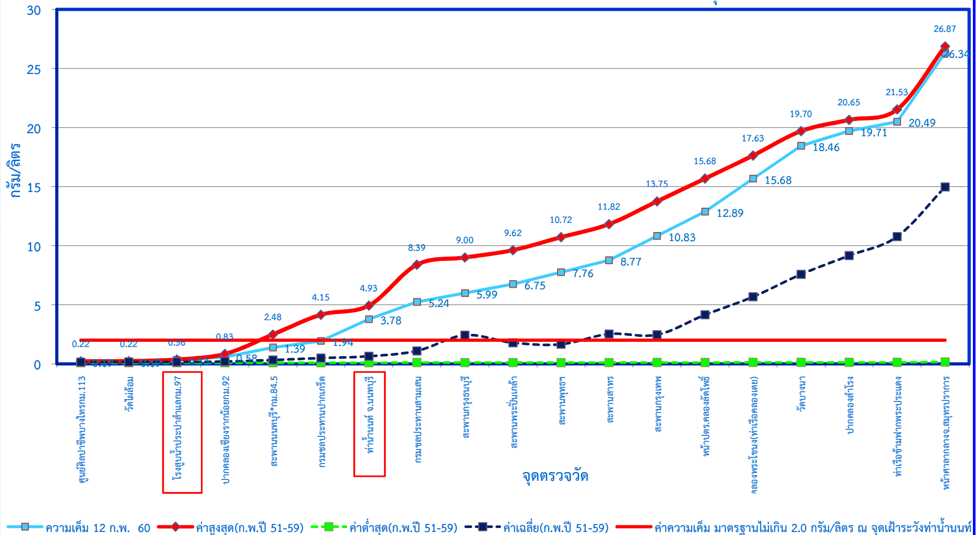
กราฟแสดงค่าความเค็มในแม่น้ำเจ้าพระยาตามพระราชเสาวนีย์ฯ เมื่อวันที่ 12 กุมภาพันธ์ 2560
