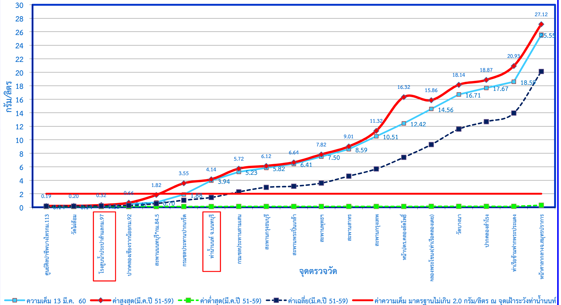
กราฟแสดงค่าความเค็มในแม่น้ำเจ้าพระยาตามพระราชเสาวนีย์ฯ เมื่อวันที่ 13 มีนาคม 2560
