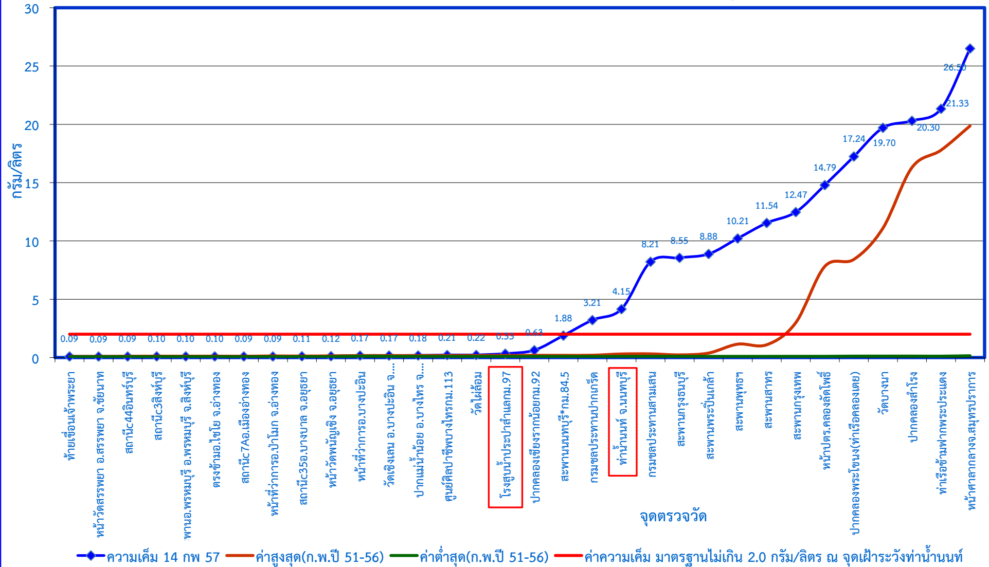
กราฟแสดงค่าความเค็มในแม่น้ำเจ้าพระยาตามพระราชเสาวนีย์ฯ เมื่อวันที่ ๑๔ กุมภาพันธ์ ๒๕๕๗
