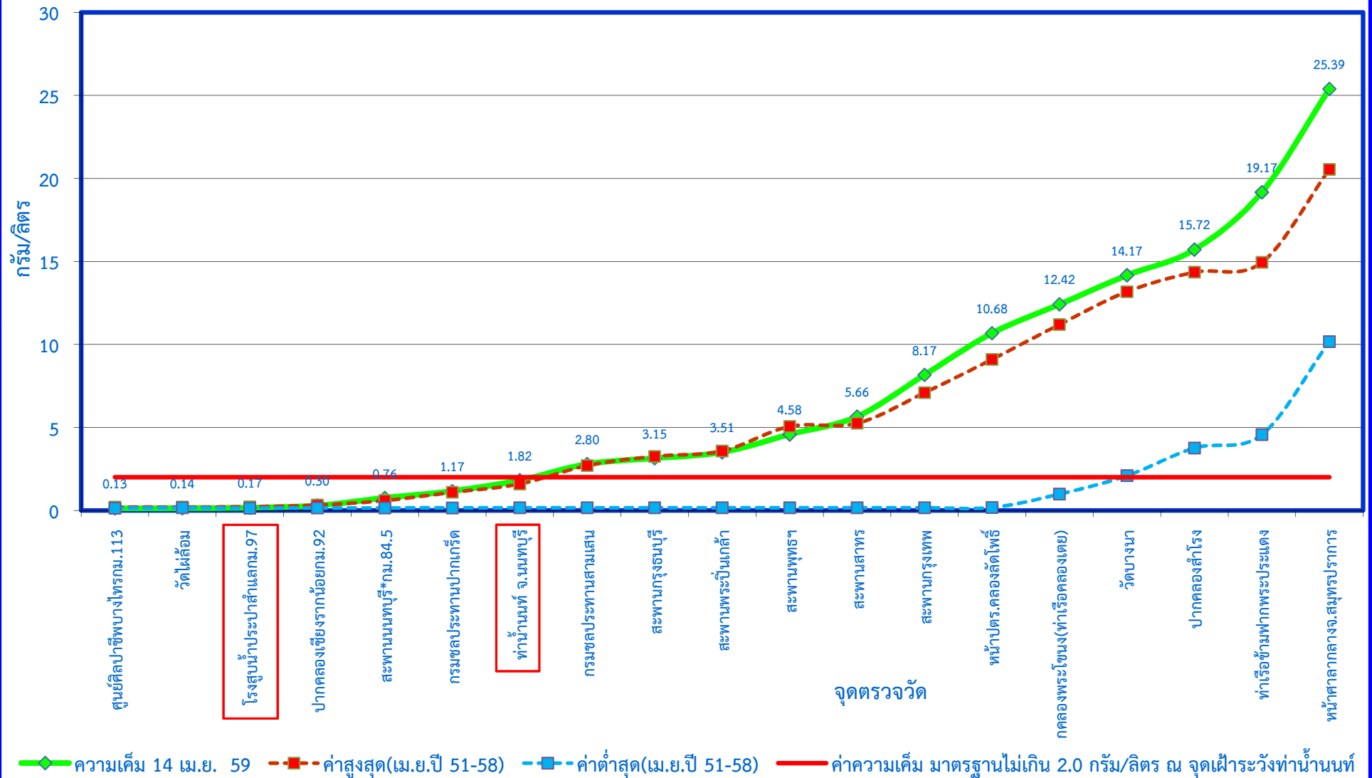
กราฟแสดงค่าความเค็มในแม่น้ำเจ้าพระยาตามพระราชเสาวนีย์ฯ เมื่อวันที่ 14 เมษายน 2559
