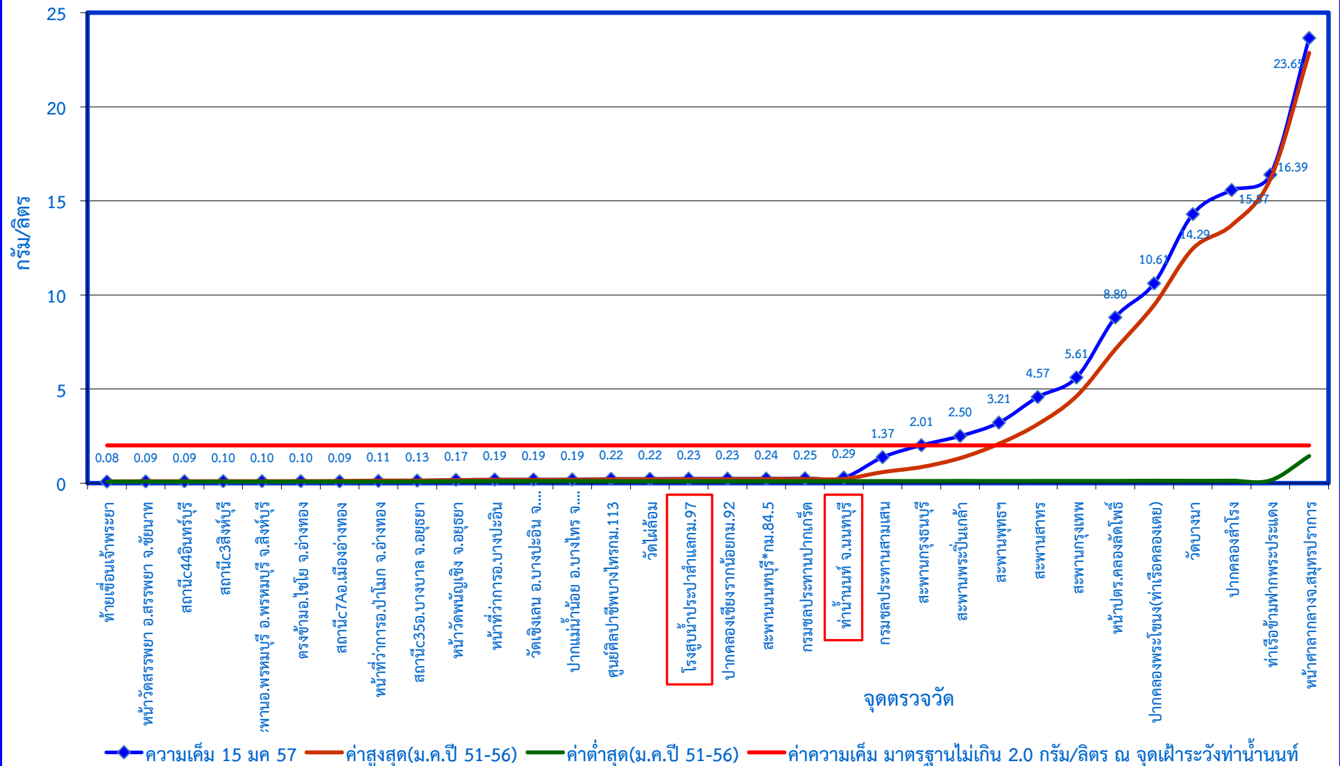
กราฟแสดงค่าความเค็มในแม่น้ำเจ้าพระยาตามพระราชเสาวนีย์ฯ เมื่อวันที่ ๑๕ มกราคม ๒๕๕๗
