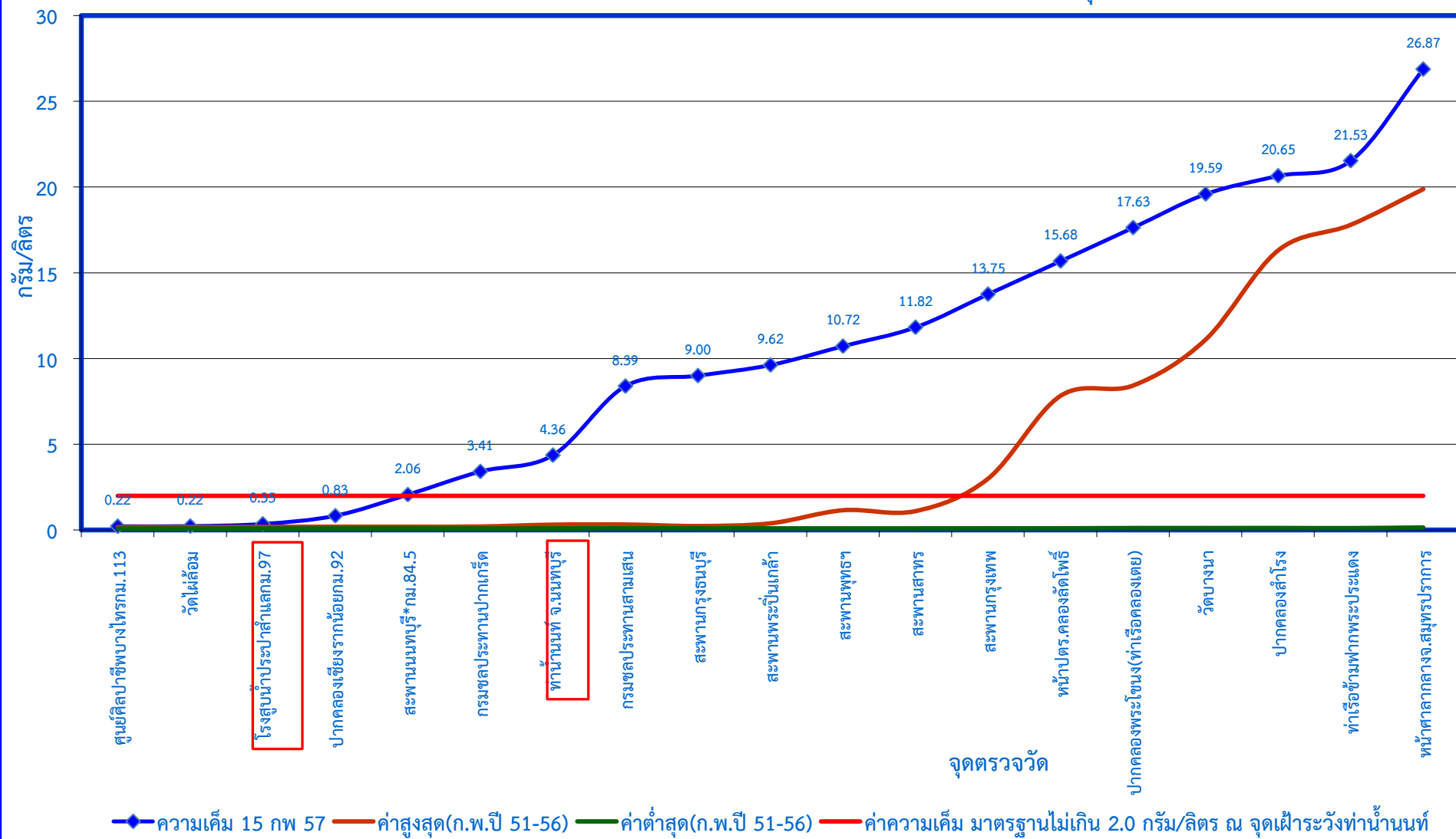
กราฟแสดงค่าความเค็มในแม่น้ำเจ้าพระยาตามพระราชเสาวนีย์ฯ เมื่อวันที่ ๑๕ กุมภาพันธ์ ๒๕๕๗
