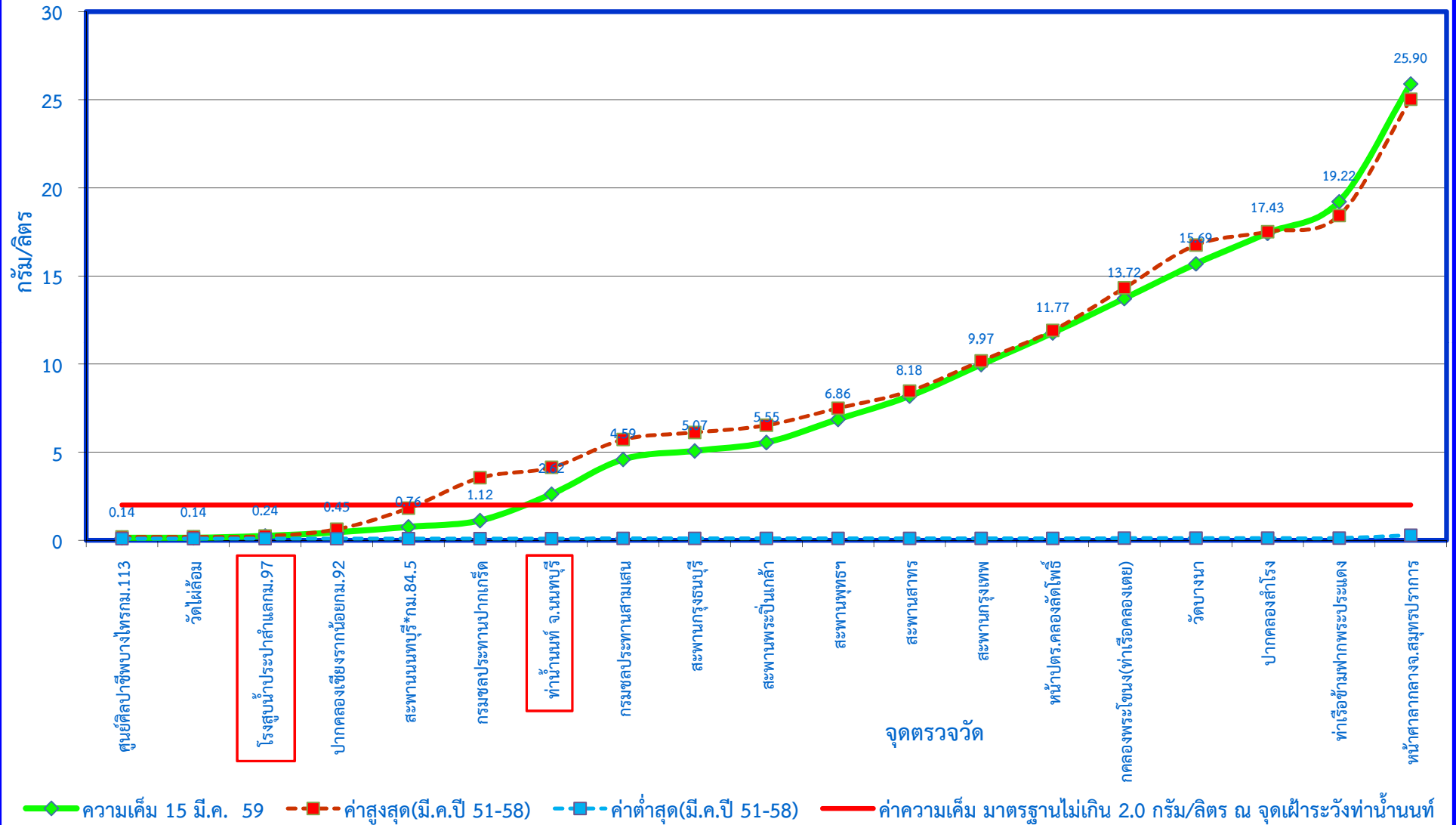
กราฟแสดงค่าความเค็มในแม่น้ำเจ้าพระยาตามพระราชเสาวนีย์ฯ เมื่อวันที่ 15 มีนาคม 2559
