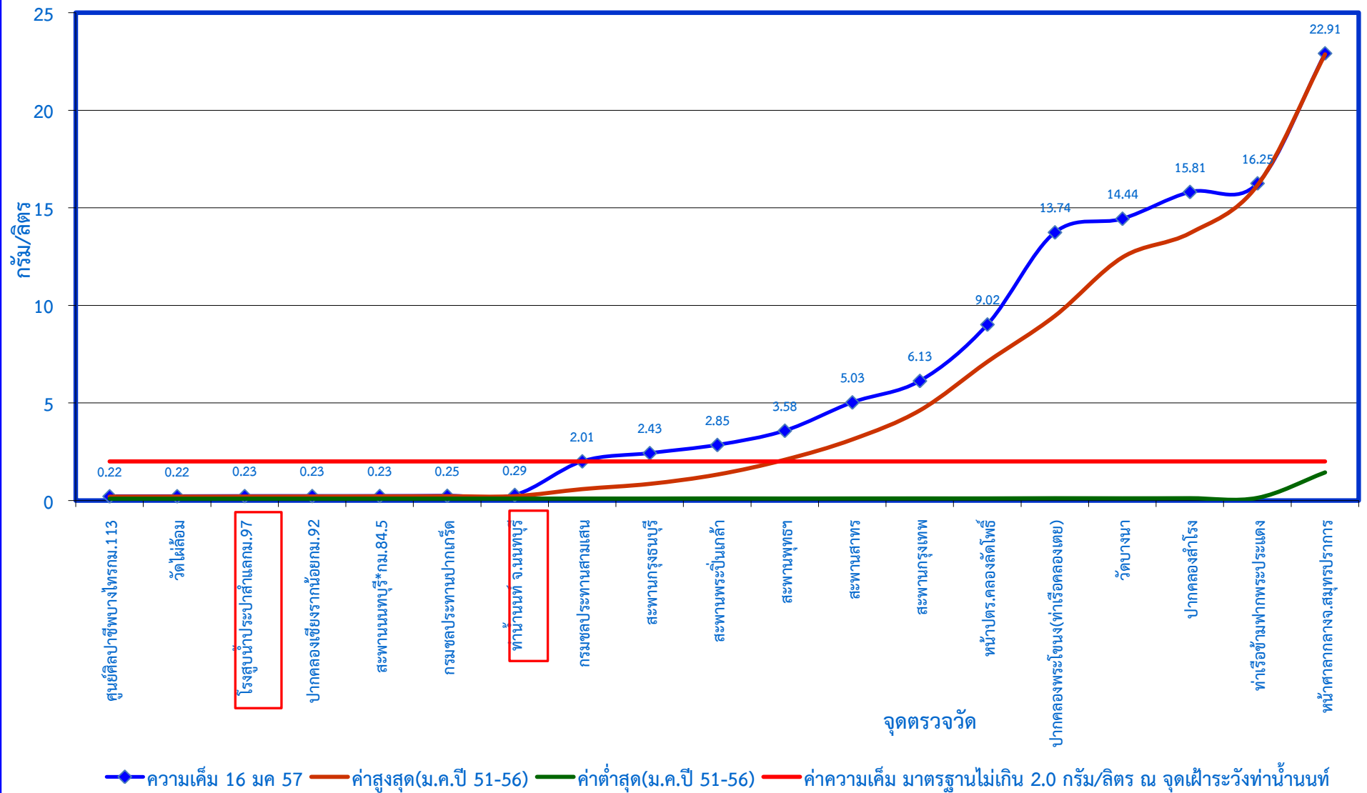
กราฟแสดงค่าความเค็มในแม่น้ำเจ้าพระยาตามพระราชเสาวนีย์ฯ เมื่อวันที่ ๑๖ มกราคม ๒๕๕๗
