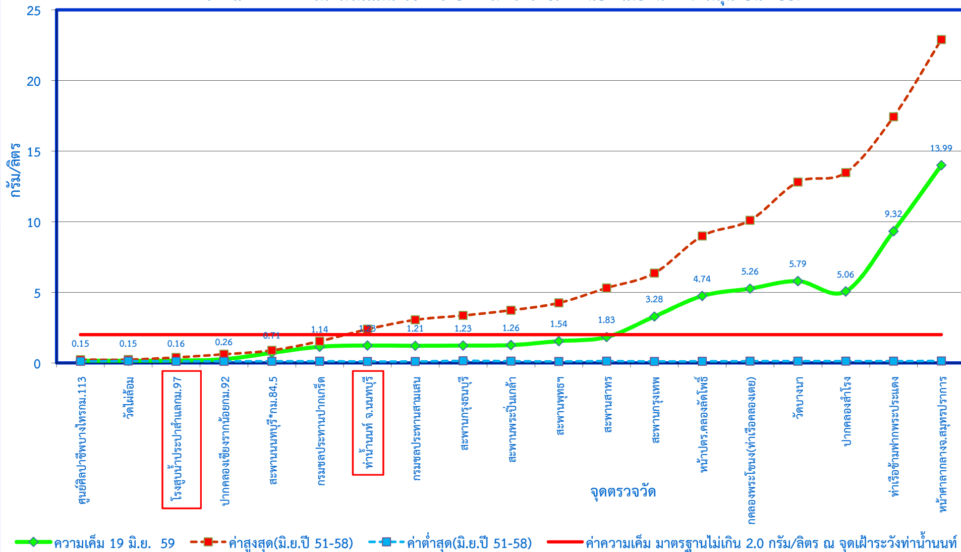
กราฟแสดงค่าความเค็มในแม่น้ำเจ้าพระยาตามพระราชเสาวนีย์ฯ เมื่อวันที่ 19 มิถุนายน 2559
