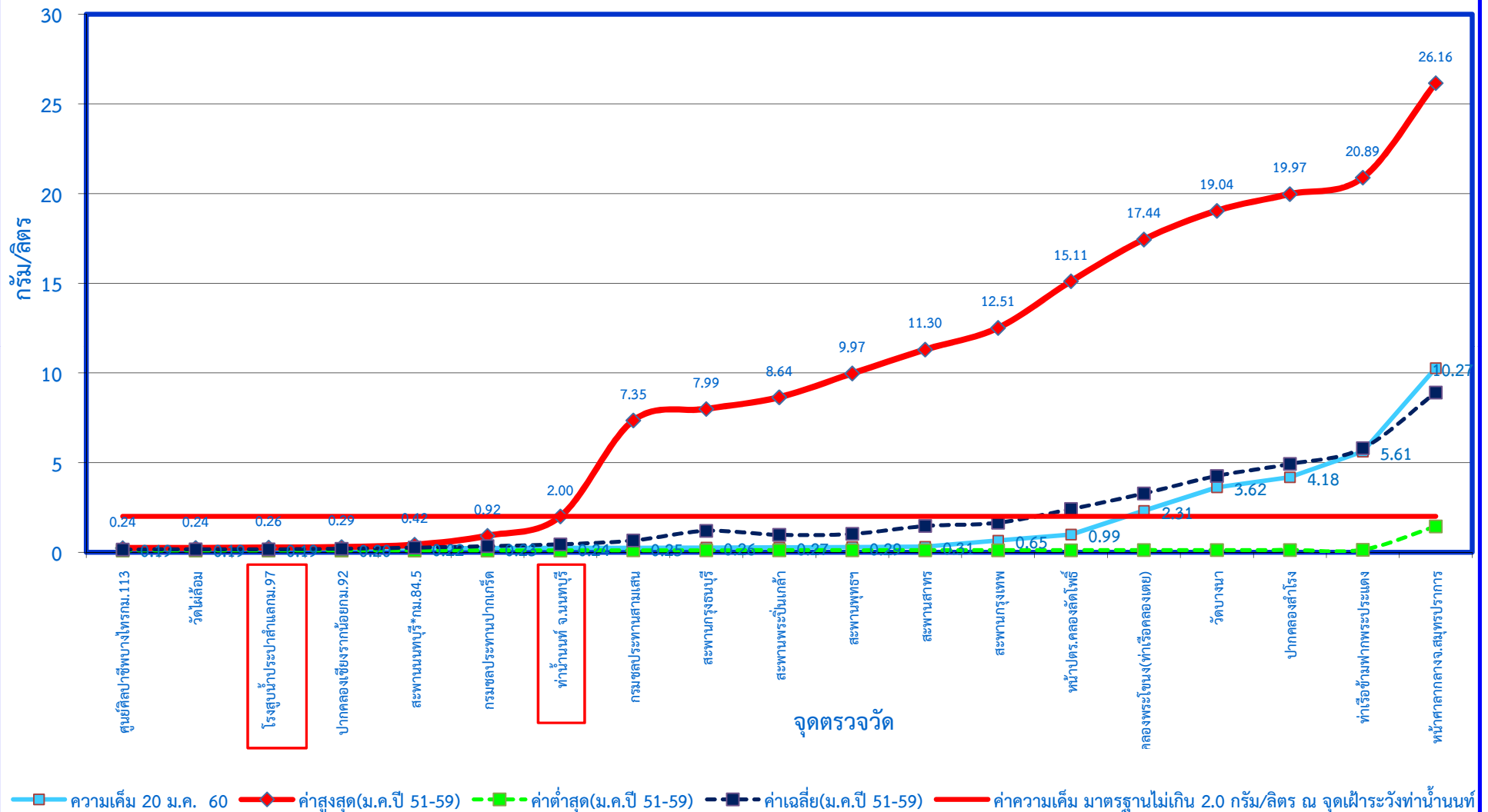
กราฟแสดงค่าความเค็มในแม่น้ำเจ้าพระยาตามพระราชเสาวนีย์ฯ เมื่อวันที่ 20 มกราคม 2560
