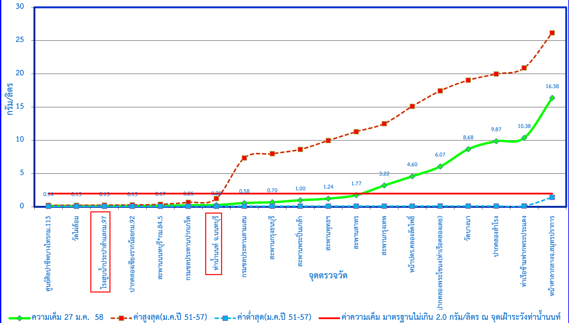
กราฟแสดงค่าความเค็มในแม่น้ำเจ้าพระยาตามพระราชเสาวนีย์ฯ เมื่อวันที่ 27 มกราคม 2558
