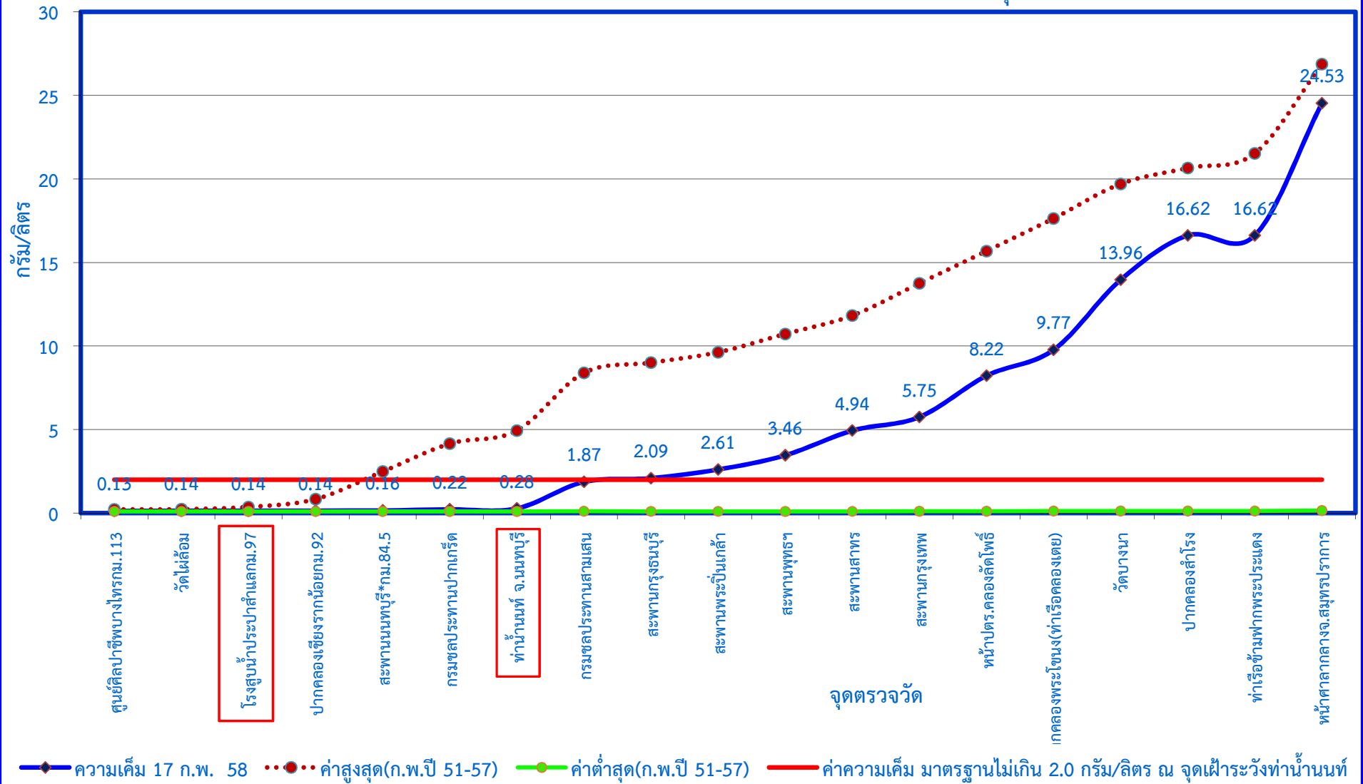
กราฟแสดงค่าความเค็มในแม่น้ำเจ้าพระยาตามพระราชเสาวนีย์ฯ เมื่อวันที่ 17 กุมภาพันธ์ 2558
