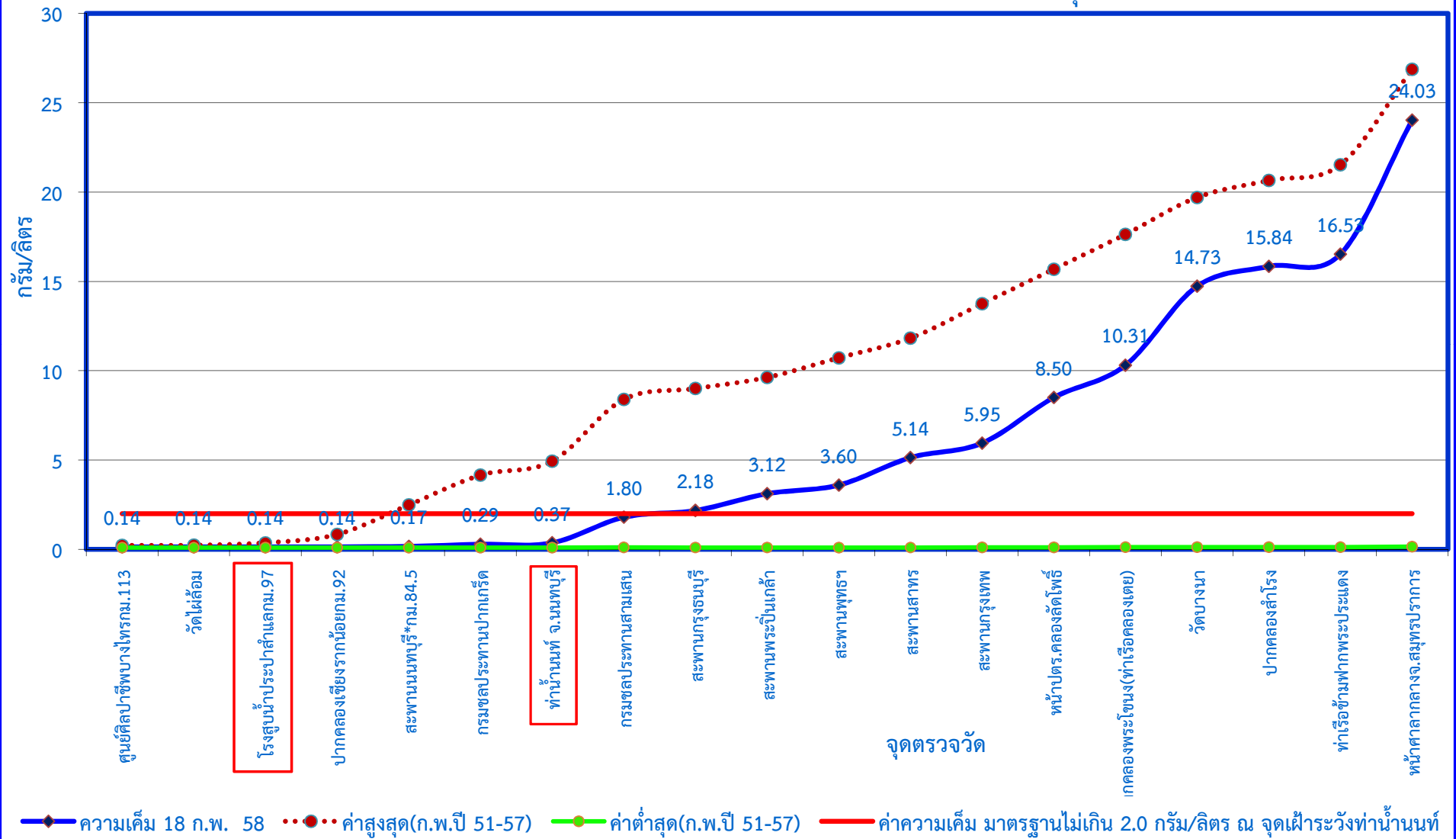
กราฟแสดงค่าความเค็มในแม่น้ำเจ้าพระยาตามพระราชเสาวนีย์ฯ เมื่อวันที่ 18 กุมภาพันธ์ 2558
