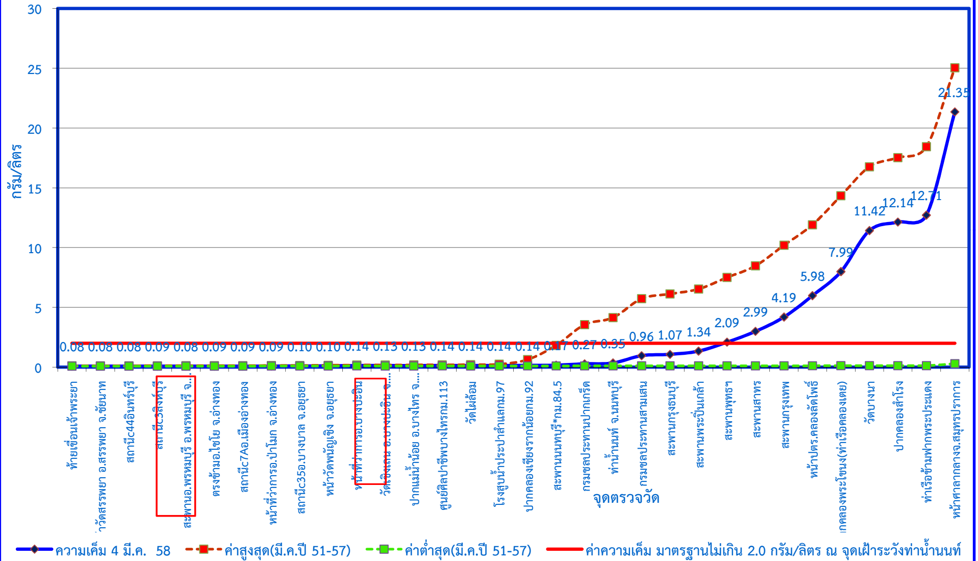
กราฟแสดงค่าความเค็มในแม่น้ำเจ้าพระยาตามพระราชเสาวนีย์ฯ เมื่อวันที่ 4 มีนาคม 2558
