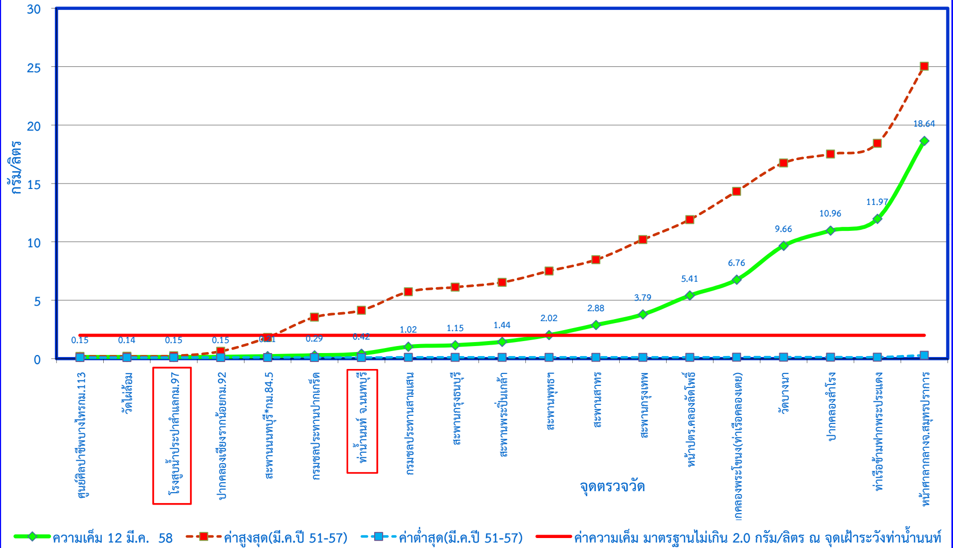
กราฟแสดงค่าความเค็มในแม่น้ำเจ้าพระยาตามพระราชเสาวนีย์ฯ เมื่อวันที่ 12 มีนาคม 2558
