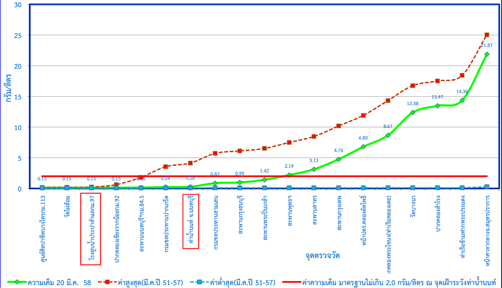
กราฟแสดงค่าความเค็มในแม่น้ำเจ้าพระยาตามพระราชเสาวนีย์ฯ เมื่อวันที่ 20 มีนาคม 2558
