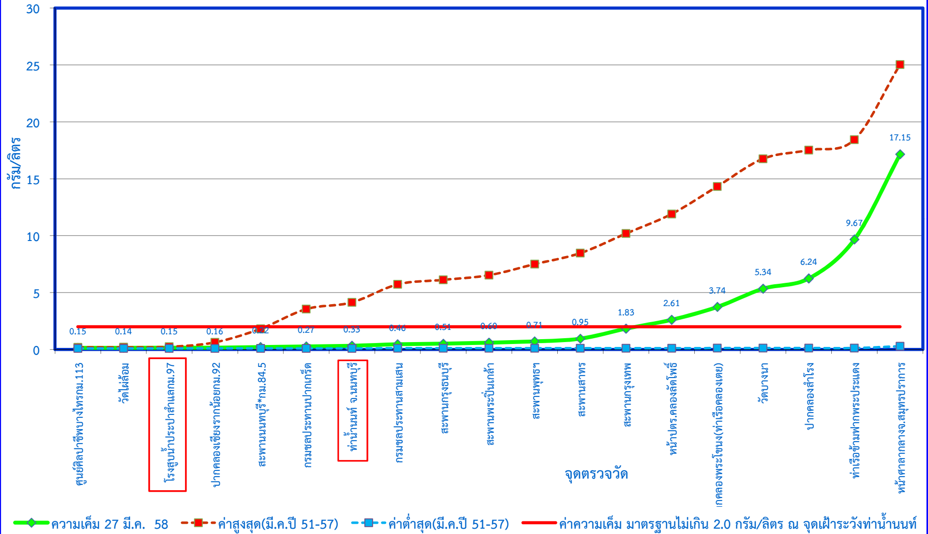
กราฟแสดงค่าความเค็มในแม่น้ำเจ้าพระยาตามพระราชเสาวนีย์ฯ เมื่อวันที่ 27 มีนาคม 2558
