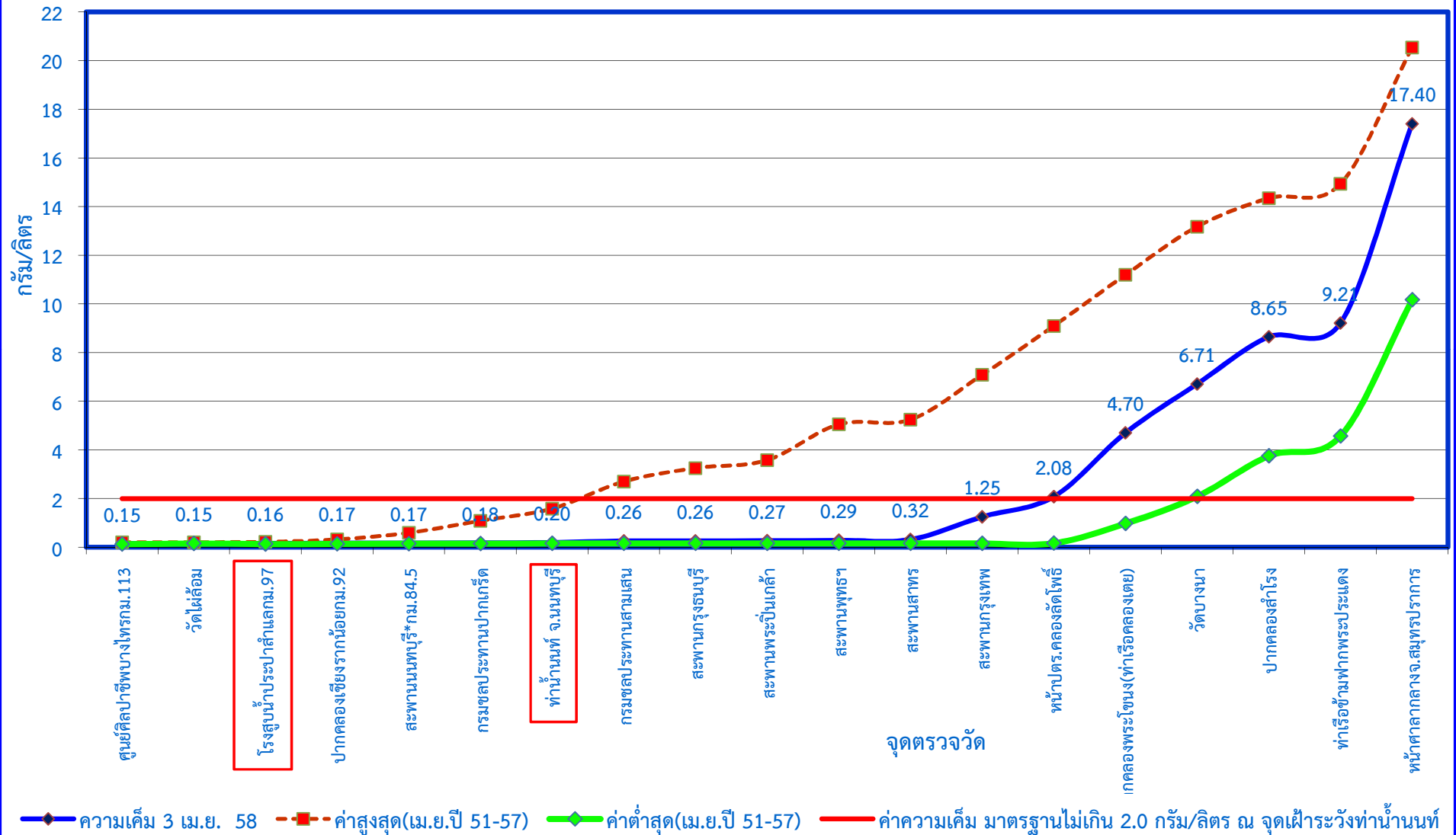
กราฟแสดงค่าความเค็มในแม่น้ำเจ้าพระยาตามพระราชเสาวนีย์ฯ เมื่อวันที่ 3 เมษายน 2558
