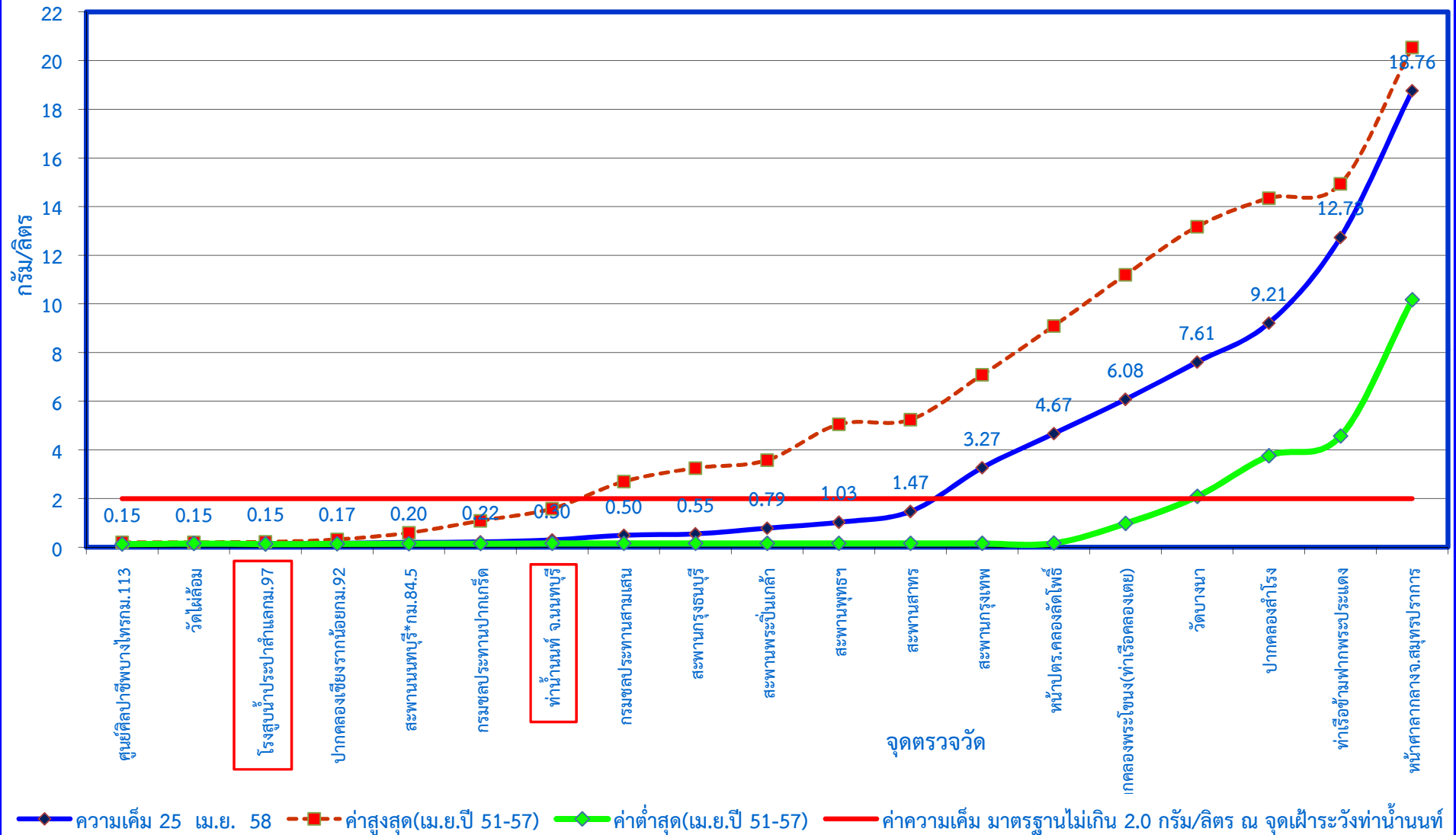
กราฟแสดงค่าความเค็มในแม่น้ำเจ้าพระยาตามพระราชเสาวนีย์ฯ เมื่อวันที่ 25 เมษายน 2558
