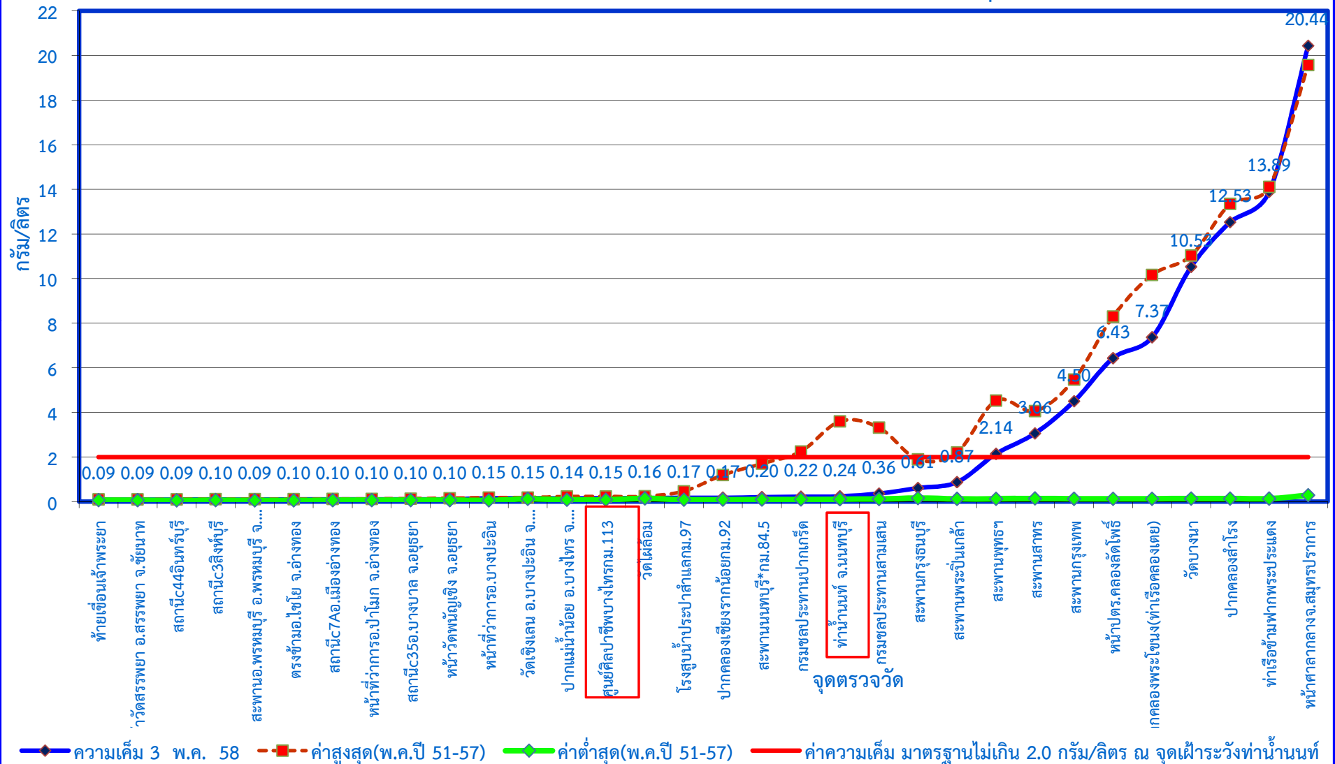
กราฟแสดงค่าความเค็มในแม่น้ำเจ้าพระยาตามพระราชเสาวนีย์ฯ เมื่อวันที่ 3 พฤษภาคม 2558
