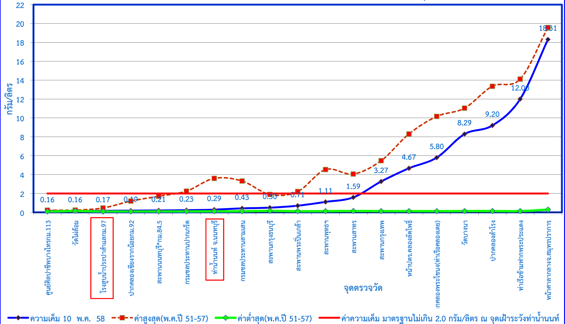
กราฟแสดงค่าความเค็มในแม่น้ำเจ้าพระยาตามพระราชเสาวนีย์ฯ เมื่อวันที่ 10 พฤษภาคม 2558
