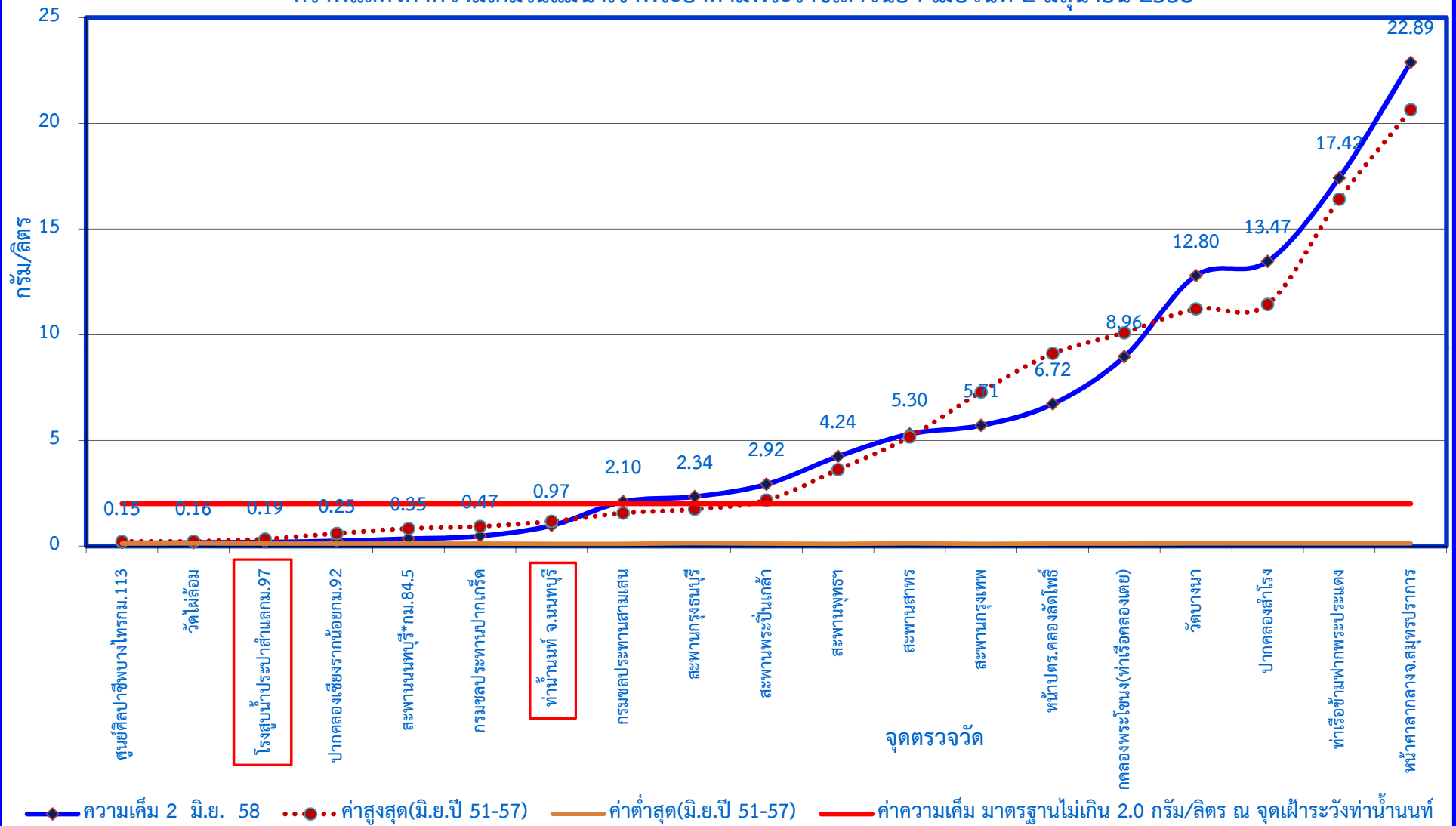
กราฟแสดงค่าความเค็มในแม่น้ำเจ้าพระยาตามพระราชเสาวนีย์ฯ เมื่อวันที่ 2 มิถุนายน 2558
