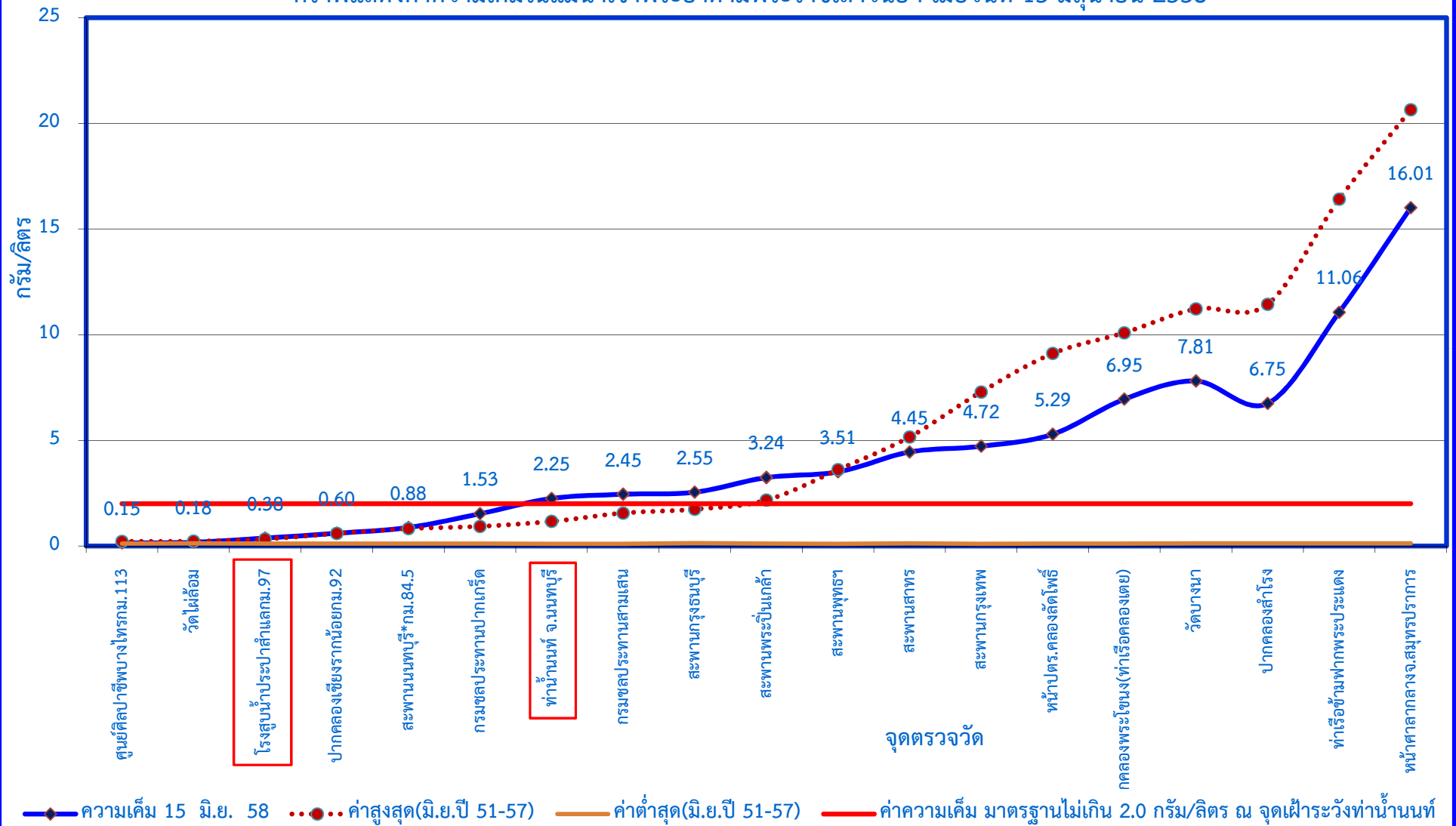
กราฟแสดงค่าความเค็มในแม่น้ำเจ้าพระยาตามพระราชเสาวนีย์ฯ เมื่อวันที่ 15 มิถุนายน 2558
