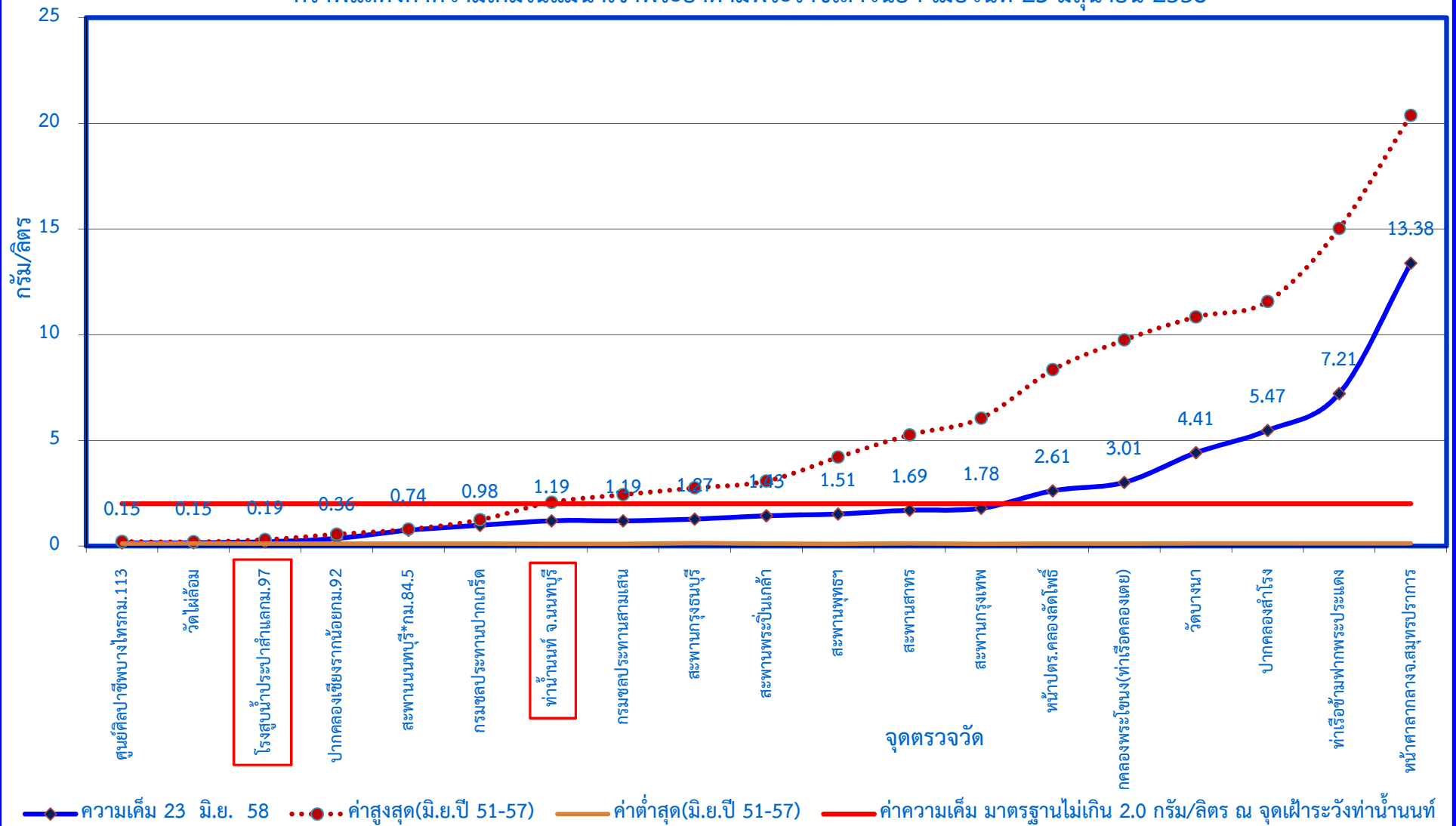
กราฟแสดงค่าความเค็มในแม่น้ำเจ้าพระยาตามพระราชเสาวนีย์ฯ เมื่อวันที่ 23 มิถุนายน 2558
