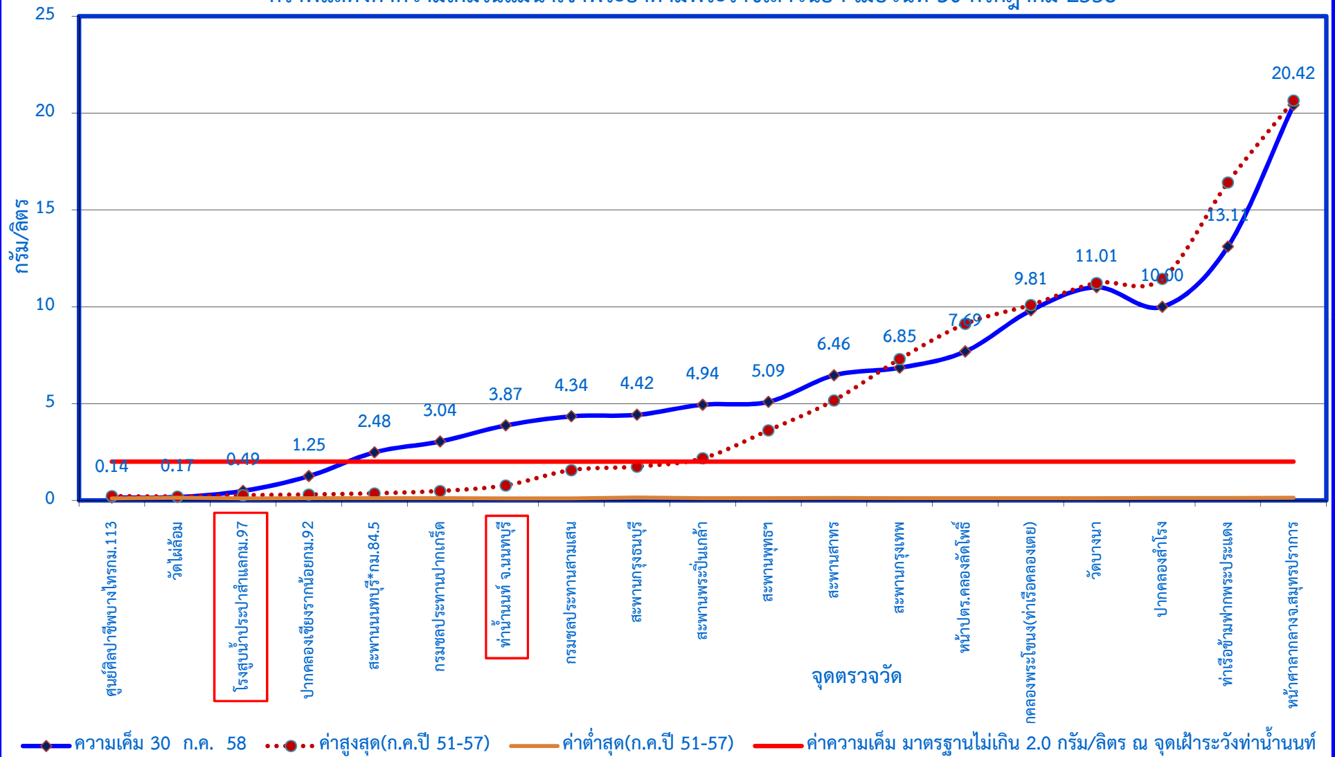
กราฟแสดงค่าความเค็มในแม่น้ำเจ้าพระยาตามพระราชเสาวนีย์ฯ เมื่อวันที่ 30 กรกฎาคม 2558
