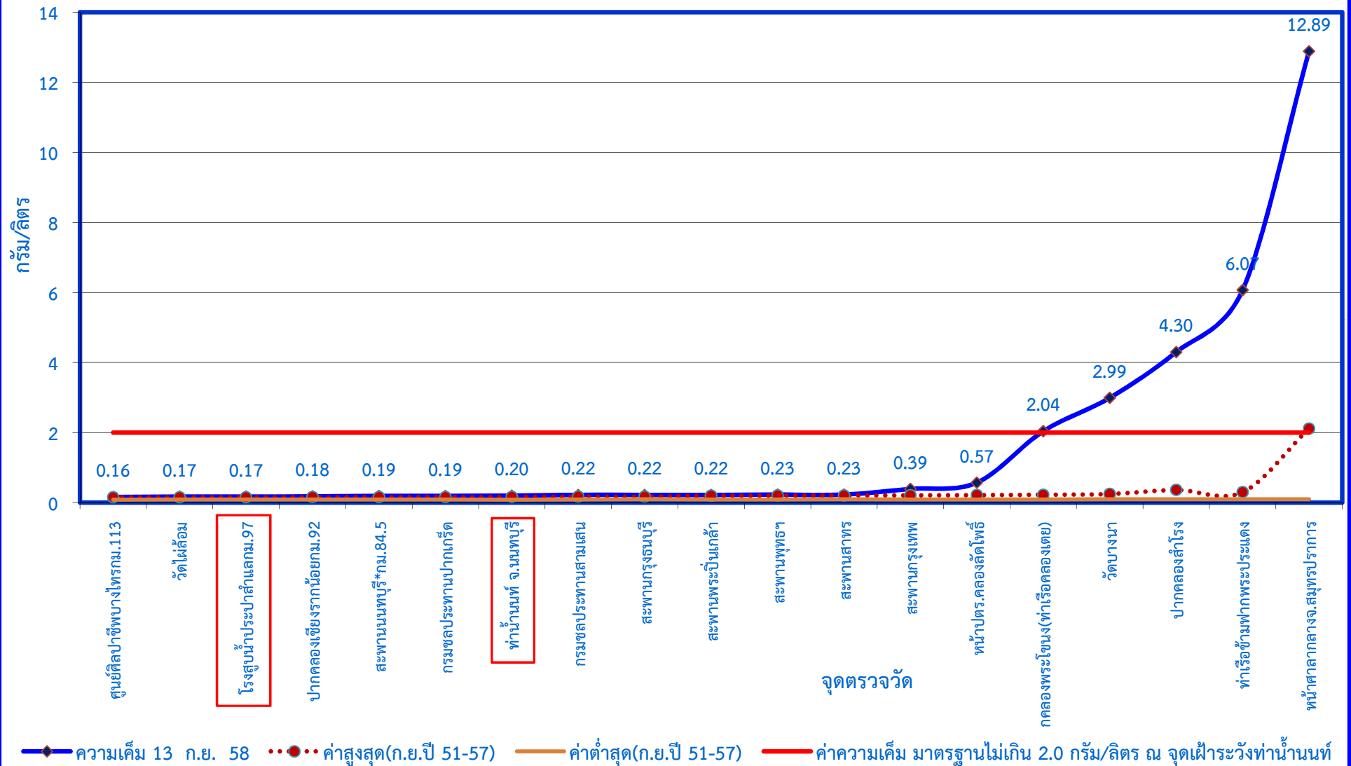
กราฟแสดงค่าความเค็มในแม่น้ำเจ้าพระยาตามพระราชเสาวนีย์ฯ เมื่อวันที่ 13 กันยายน 2558
