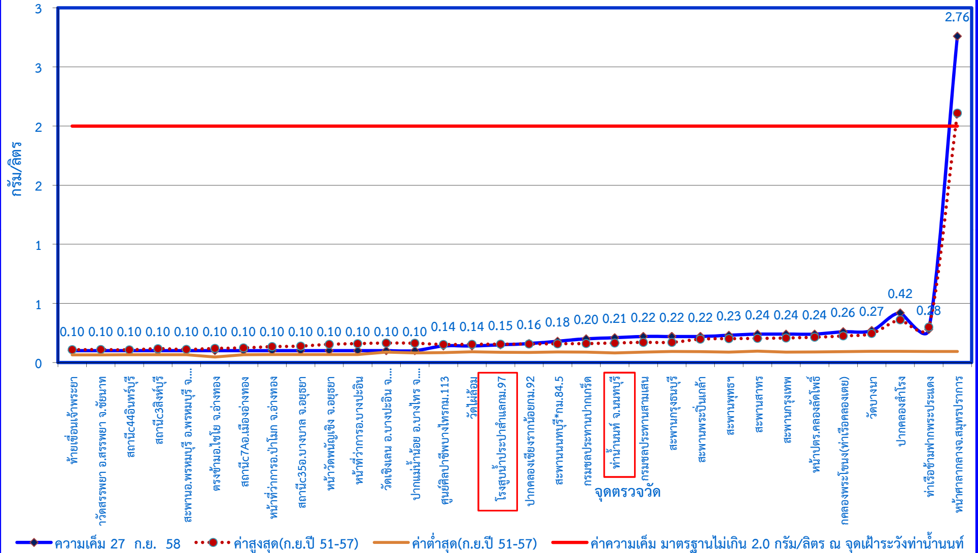
กราฟแสดงค่าความเค็มในแม่น้ำเจ้าพระยาตามพระราชเสาวนีย์ฯ เมื่อวันที่ 27 กันยายน 2558
