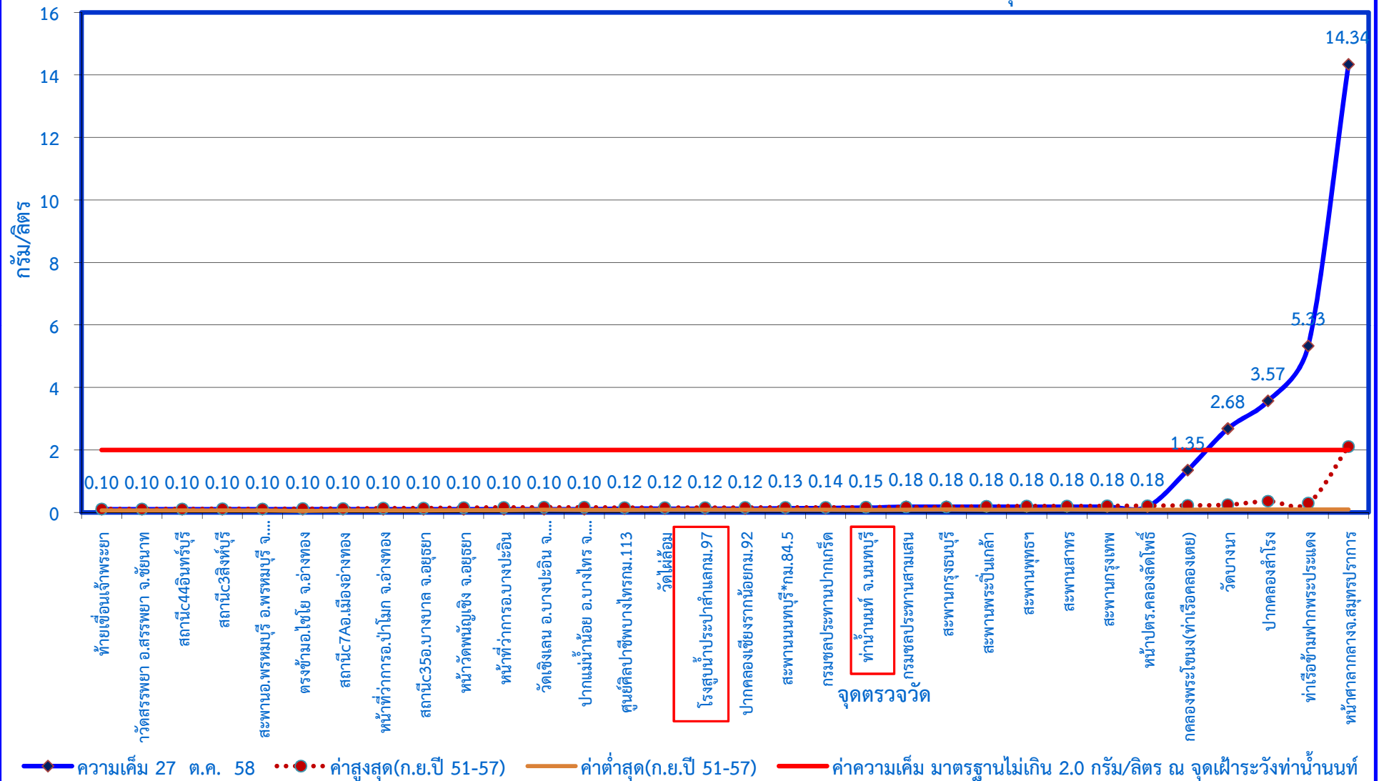
กราฟแสดงค่าความเค็มในแม่น้ำเจ้าพระยาตามพระราชเสาวนีย์ฯ เมื่อวันที่ 27 ตุลาคม 2558
