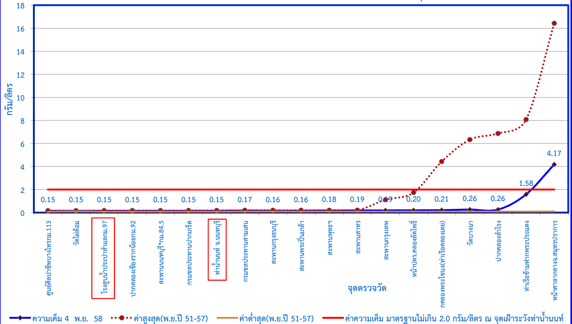
กราฟแสดงค่าความเค็มในแม่น้ำเจ้าพระยาตามพระราชเสาวนีย์ฯ เมื่อวันที่ 4 พฤศจิกายน 2558
