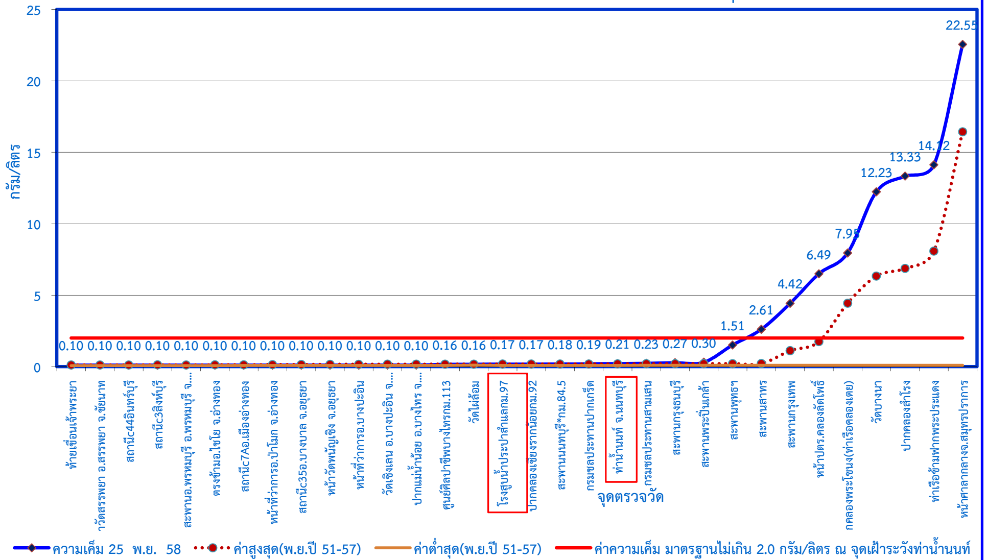
กราฟแสดงค่าความเค็มในแม่น้ำเจ้าพระยาตามพระราชเสาวนีย์ฯ เมื่อวันที่ 25 พฤศจิกายน 2558
