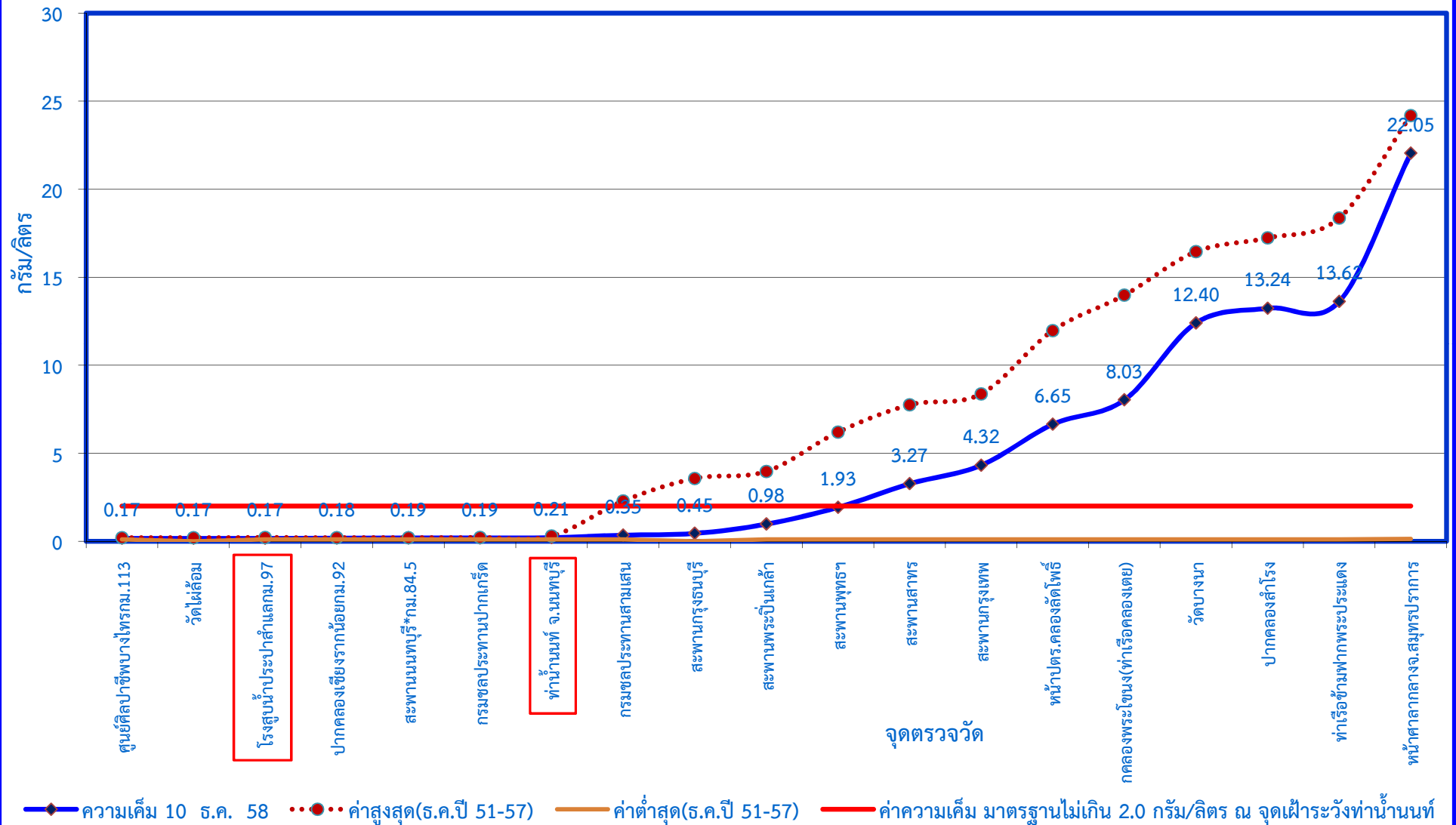
กราฟแสดงค่าความเค็มในแม่น้ำเจ้าพระยาตามพระราชเสาวนีย์ฯ เมื่อวันที่ 10 ธันวาคม 2558
