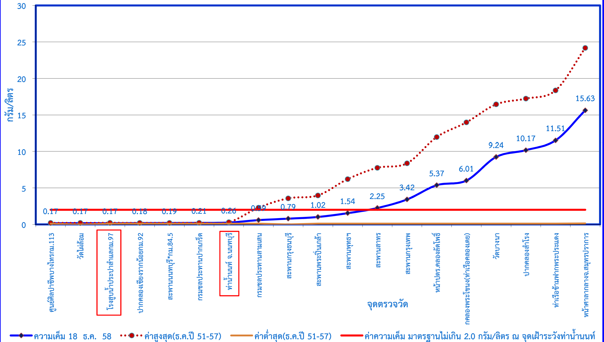
กราฟแสดงค่าความเค็มในแม่น้ำเจ้าพระยาตามพระราชเสาวนีย์ฯ เมื่อวันที่ 18 ธันวาคม 2558
