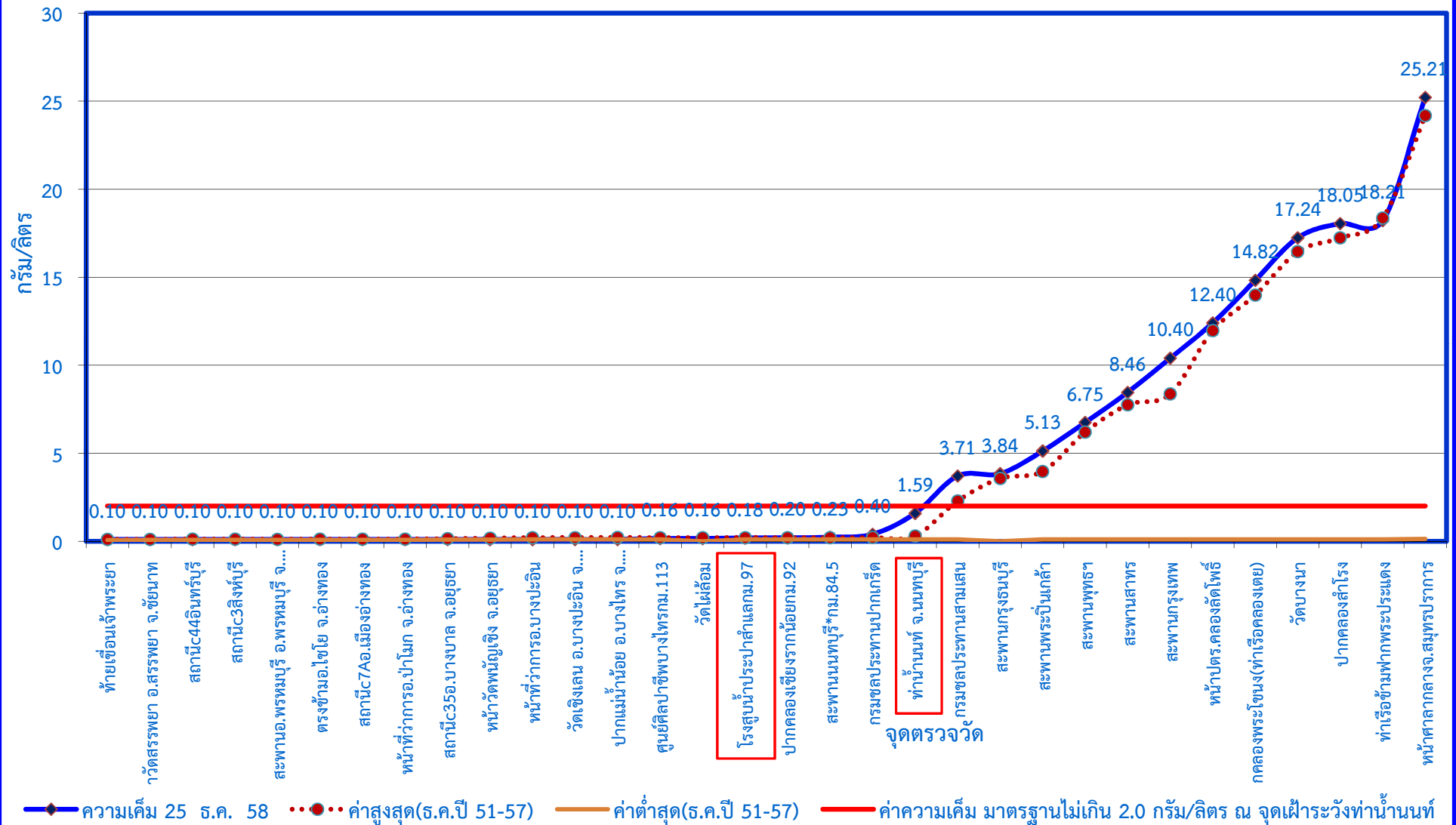
กราฟแสดงค่าความเค็มในแม่น้ำเจ้าพระยาตามพระราชเสาวนีย์ฯ เมื่อวันที่ 25 ธันวาคม 2558
