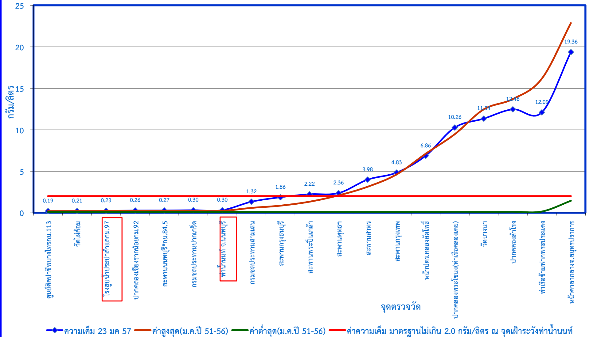
กราฟแสดงค่าความเค็มในแม่น้ำเจ้าพระยาตามพระราชเสาวนีย์ฯ เมื่อวันที่ ๒๓ มกราคม ๒๕๕๗
