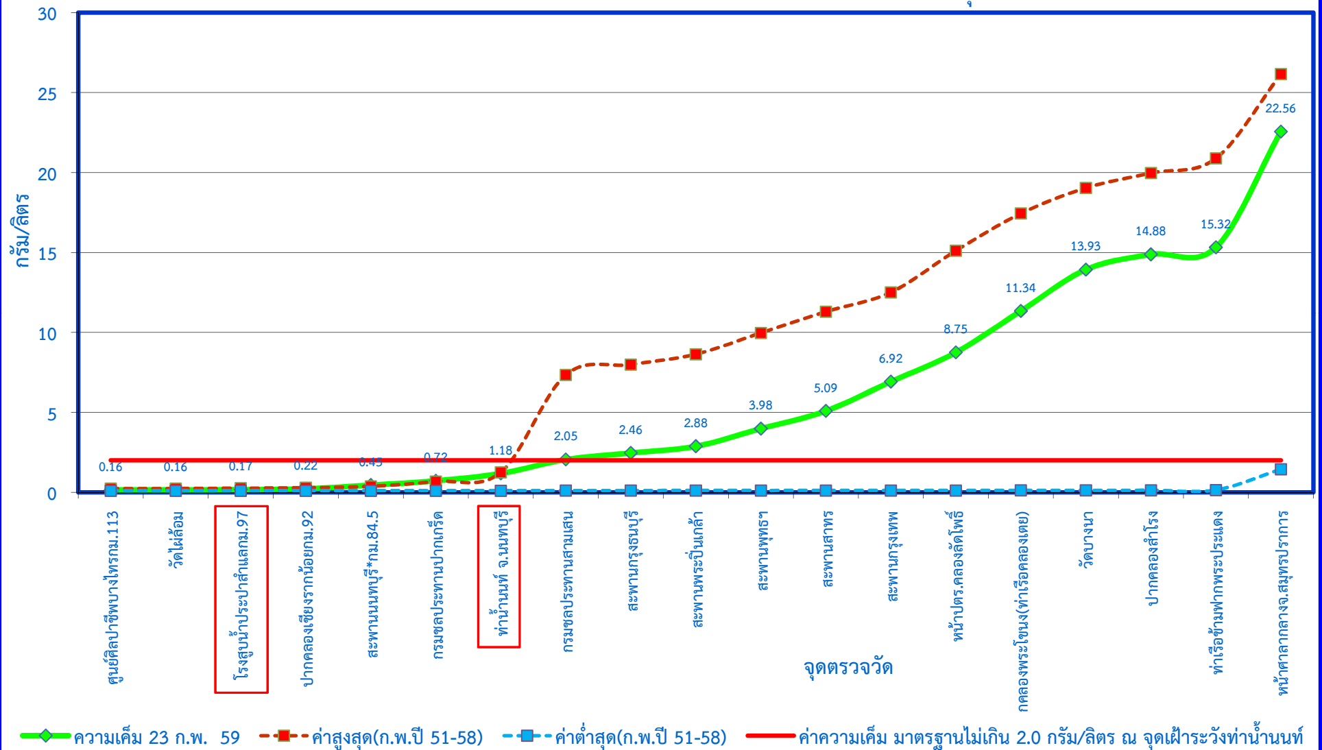
กราฟแสดงค่าความเค็มในแม่น้ำเจ้าพระยาตามพระราชเสาวนีย์ฯ เมื่อวันที่ 23 กุมภาพันธ์ 2559
