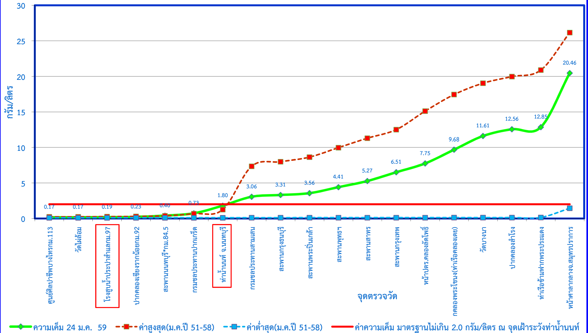
กราฟแสดงค่าความเค็มในแม่น้ำเจ้าพระยาตามพระราชเสาวนีย์ฯ เมื่อวันที่ 24 มกราคม 2559
