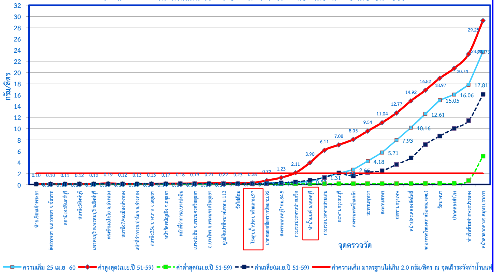
กราฟแสดงค่าความเค็มในแม่น้ำเจ้าพระยาตามพระราชเสาวนีย์ฯ เมื่อวันที่ 25 เมษายน 2560
