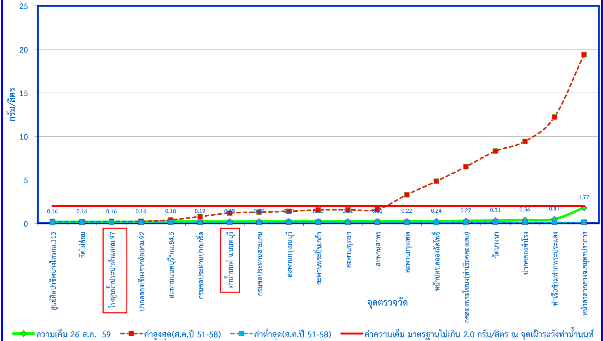
กราฟแสดงค่าความเค็มในแม่น้ำเจ้าพระยาตามพระราชเสาวนีย์ฯ เมื่อวันที่ 26 สิงหาคม 2559
