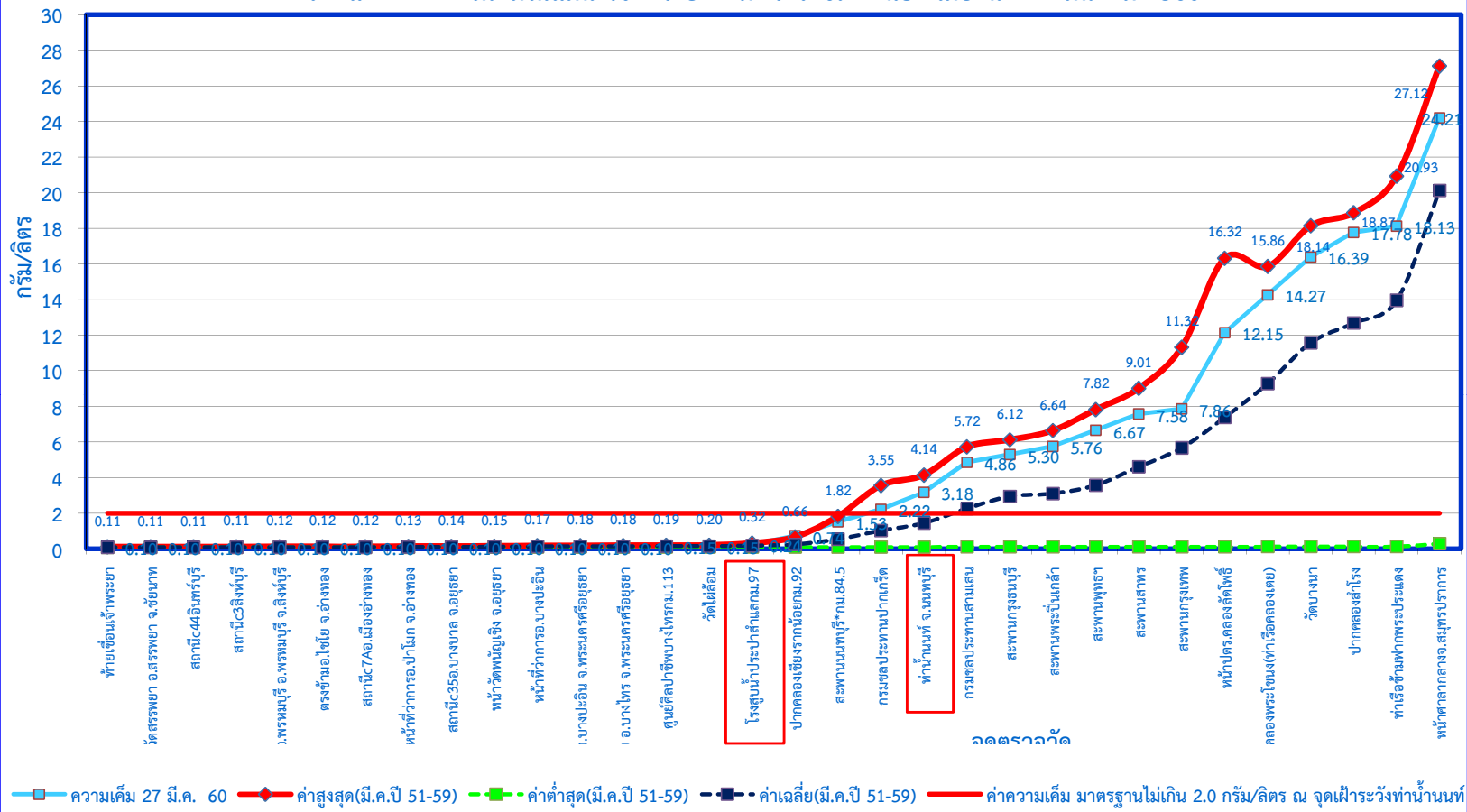
กราฟแสดงค่าความเค็มในแม่น้ำเจ้าพระยาตามพระราชเสาวนีย์ฯ เมื่อวันที่ 27 มีนาคม 2560
