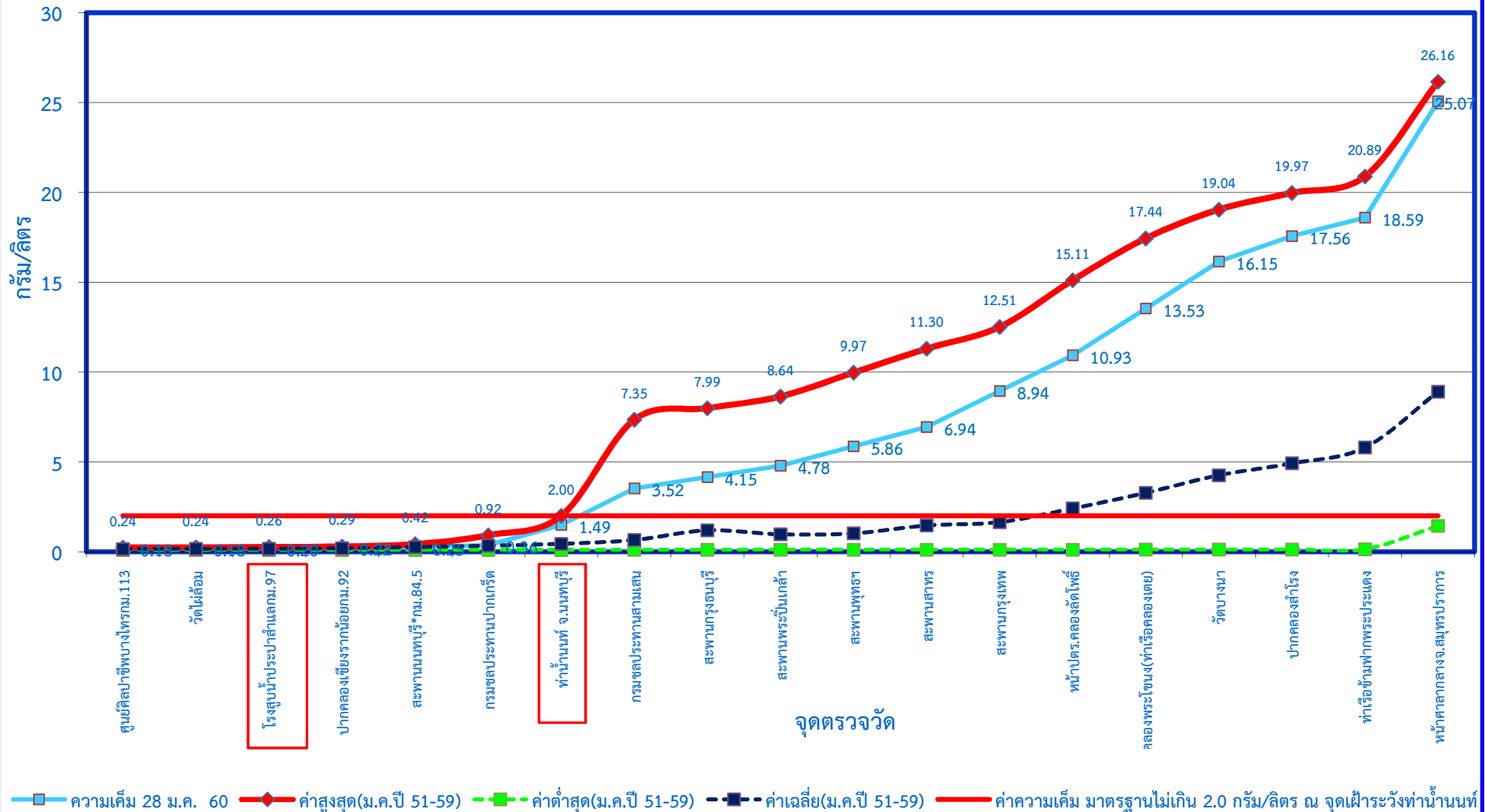
กราฟแสดงค่าความเค็มในแม่น้ำเจ้าพระยาตามพระราชเสาวนีย์ฯ เมื่อวันที่ 28 มกราคม 2560
